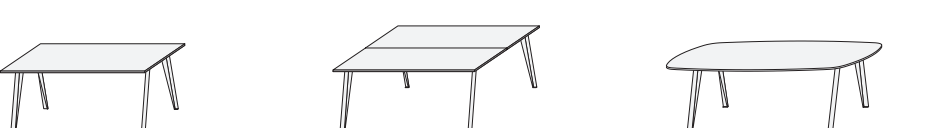
tavolo riunione conference table L.1600 P.1000 L.2200 P.1000 L.1800 P.1000 L.2400 P.1000 L.2000 P.1000 L.2600 P.1000 tavolo riunione conference table L.1600 P.1600 L.2200 P.1600 L.1800 P.1600 L.2400 P.1600 L.2000 P.1600 L.2600 P.1600 tavolo riunione sagomato shaped conference table L.2400 P.1200
