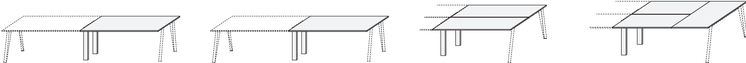
scrivania aggregabile addable desk L. 800 P.800 L.1800 P.800 L.1000 P.800 L.2000 P.800 L.1200 P.800 L.2200 P.800 L.1400 P.800 L.2400 P.800 L.1600 P.800 scrivania aggregabile addable desk L.1000 P.1000 L.2000 P.1000 L.1600 P.1000 L.2200 P.1000 L.1800 P.1000 L.2400 P.1000 nr. 2 scrivanie aggregabili nr. 2 addable desks L.1000 P.1630 L.1800 P.1630 L.1200 P.1630 L.2000 P.1630 L.1400 P.1630 L.2200 P.1630 L.1600 P.1630 L.2400 P.1630 nr. 3 scrivanie aggregabili nr. 3 addable desks L.2000 P.1630 L.2200 P.1630 L.2400 P.1630 L.2600 P.1630
