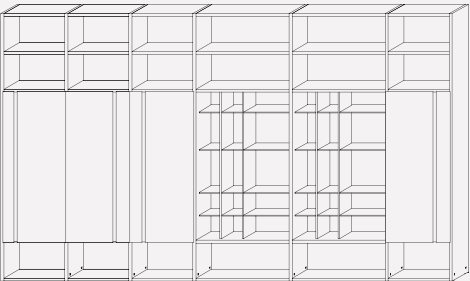
L. 4208 H. 2498 P. 346 W. 165¾” H. 98¼” D. 13½”
