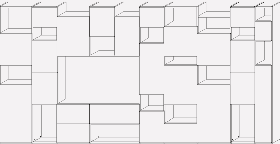
L. 4955 H. 2498 P. 346 W. 195” H. 98¼” D. 13½”
