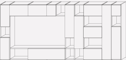
L. 3924 H. 1792 P. 346 W. 154½” H. 70½” D. 13½”
