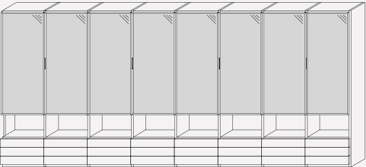
L. 4804 H. 2146 P. 442 W. 189¼” H. 84½” D. 17½”
