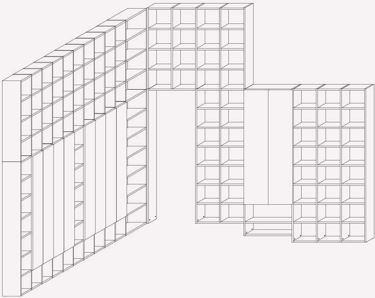
L. 5750 + 4060 H. 3996 – 2846 P. 346 W. 226½" + 159¾" H. 157¼" – 112" D. 13½"
