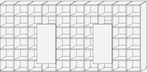
L. 4508 H. 2146 P. 442 W. 177½” H. 84½” D. 17½”
