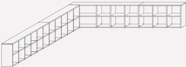
L. 5301 + 3584 H. 737 P. 346 W. 208¾" + 141" H. 29" D. 13½"
