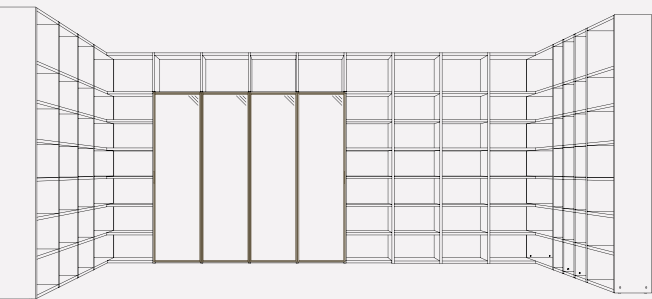
L. 6037 – 2715 – 2416 H. 2626 P. 346 W. 237¾” – 107” – 95” H. 103½” D. 13½”
