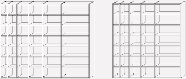
L. 2859 – 2194 H. 2390 P. 346 W. 112½” – 86¼” H. 94” D. 13½”
