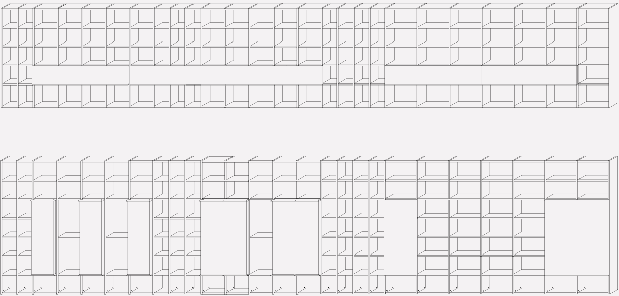
Sopra – Upper composition L. 11375 H. 1857 P. 346 W. 447¾" H. 73" D. 13½" Sotto – Bottom composition L. 11375 H. 2498 P. 346 W. 447¾" H. 98¼" D. 13½"
