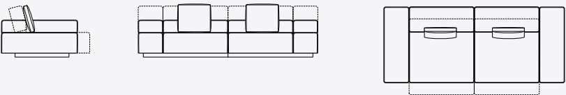
Divano 2 posti Two-seater sofa L.2760 H. 560 – 770 P.1200 – 1380 W. 107 3/4” H 22” – 30¾” D. 47¼” – 52¼
