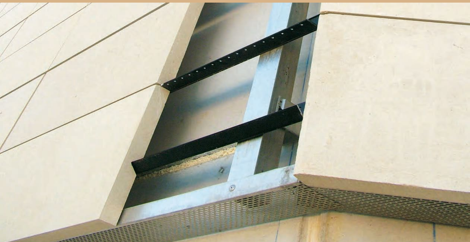
Esempio di lastre squadrate per facciate ventilate. Example of ventilated wall-cladding installed with anchoring system.
