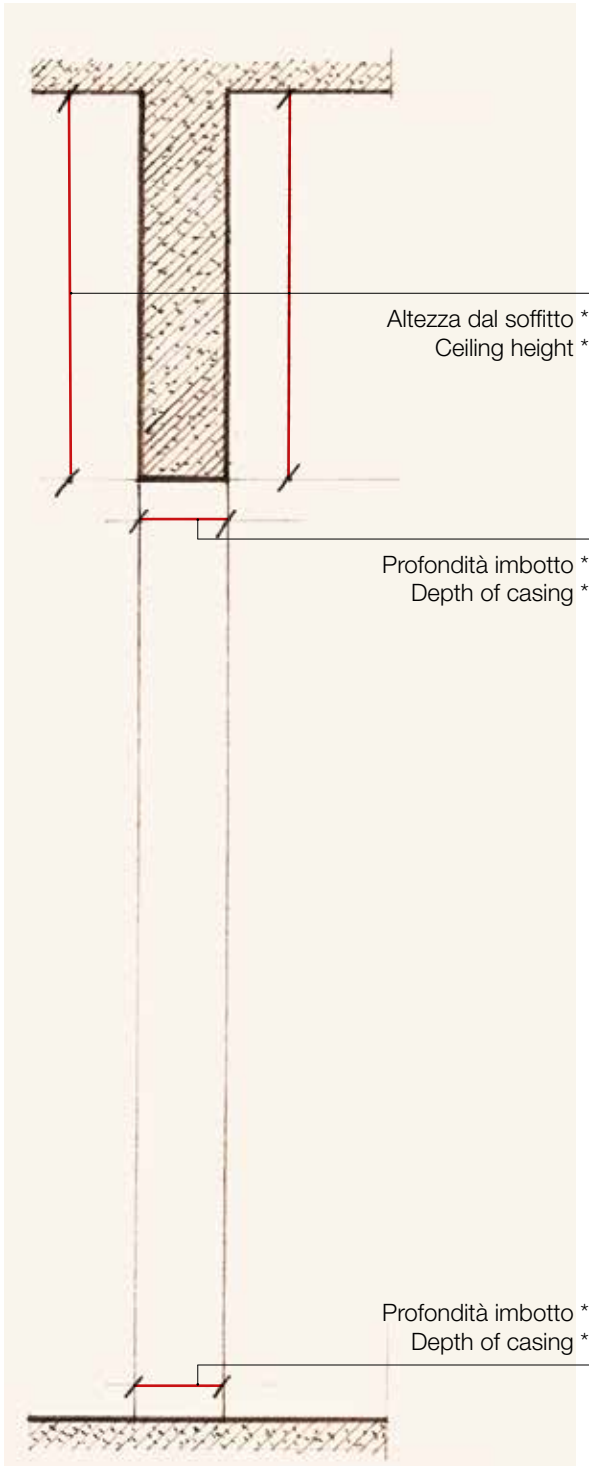
Sezione verticale -Vertical section
