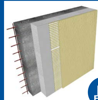
Ciclo Ferrimix: intonaco o rasatura con rete minerale antiritiro.
