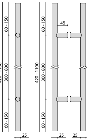
Maniglione doppio altezza mm 420/1100 Double pullhandle height 420/1100 mm
