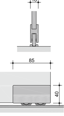
Particolare ruota Trolley detail
