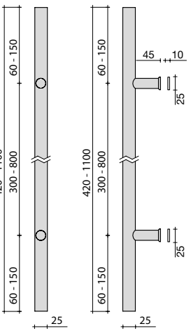
Maniglione singolo altezza mm 420/1100 Single pullhandle height 420/1100 mm
