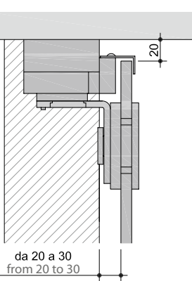
Fissaggio a soffitto Ceiling installation
