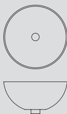
Lavabo apoyo Ø48 cm. 48 cm. countertop basin. 100170819 white/blanco 100180499 matt white/blanco mate
