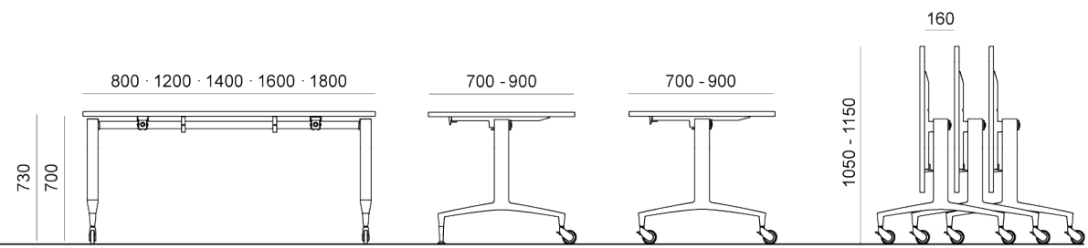
TAVOLO RIBALTABILE CON RUOTE E PIEDINI COMPENSATORI | FLIP TOP TABLE WITH CASTORS AND ADJUSTABLE GLIDES
