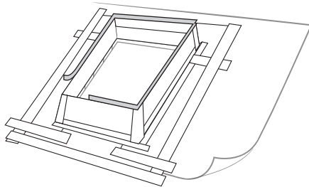
Posizionamento nastro espandente sul giunto
