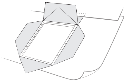
Posizionamento protezione sotto l'ultimo sormonto
