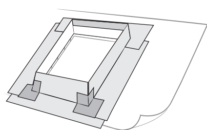
Protezione degli angoli con elementi in LDPE
