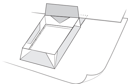
Ripiegatura dei risvolti e protezione cassonetto
