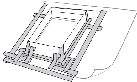
Nastratura di tutti i giunti
