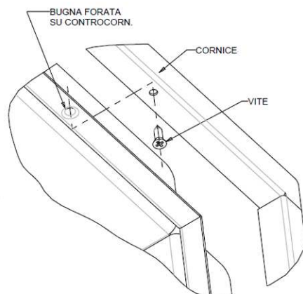
PARTIC. FISSAGGIO SUPER. CORNICE
