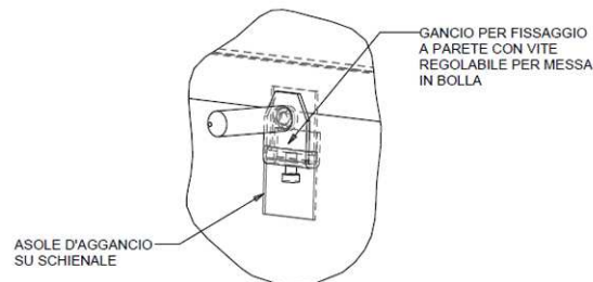
PARTIC. GANCIO DI FISSAGGIO A PARETE
