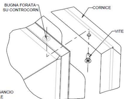
PARTIC. FISSAGGIO SUPER. CORNICE
