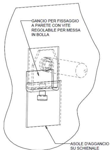
PARTIC. GANCIO DI FISSAGGIO A PARETE
