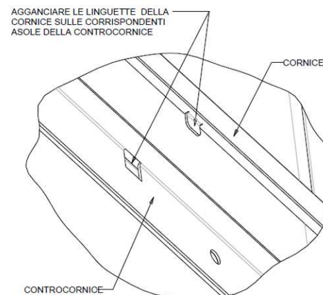
PARTIC. FISSAGGIO INFER. CORNICE
