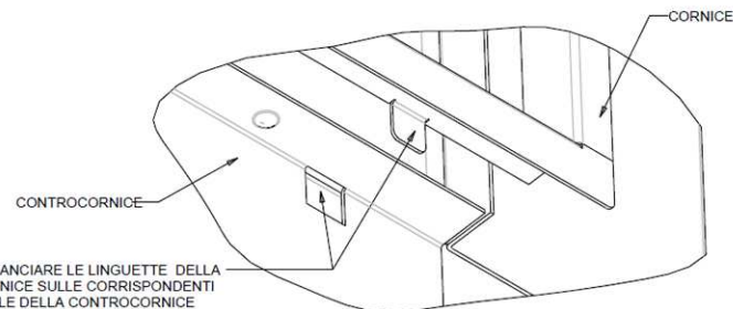
PARTIC. FISSAGGIO INFER. CORNICE
