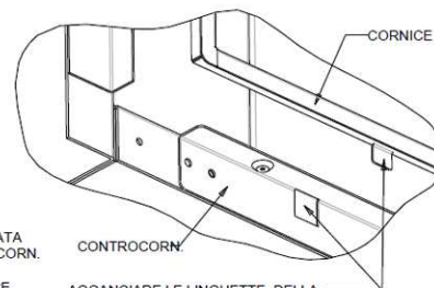
PARTIC. FISSAGGIO INFER. CORNICE
