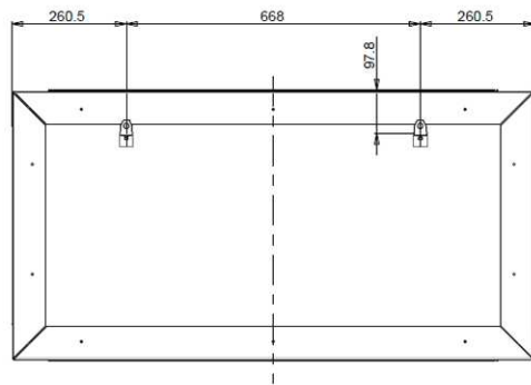
VISTA POSTERIORE
