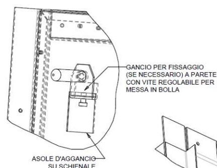
PARTIC. GANCIO DI FISSAGGIO A PARETE
