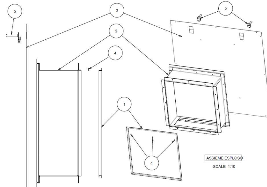
SEZIONE ESPLOSA
