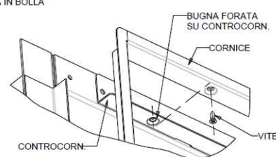
PARTIC. FISSAGGIO SUPER. CORNICE
