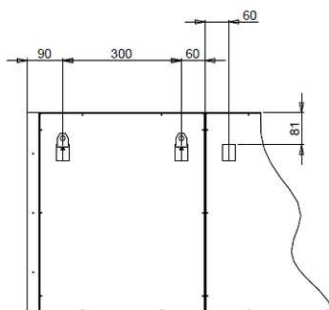
VISTA POSTERIORE PARTIC. ASOLE D'AGGANCIO SU SCHIENALE
