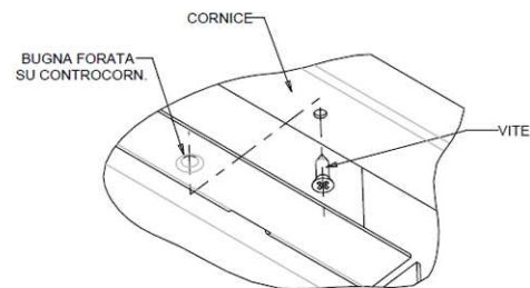
PARTIC. FISSAGGIO SUPER. CORNICE
