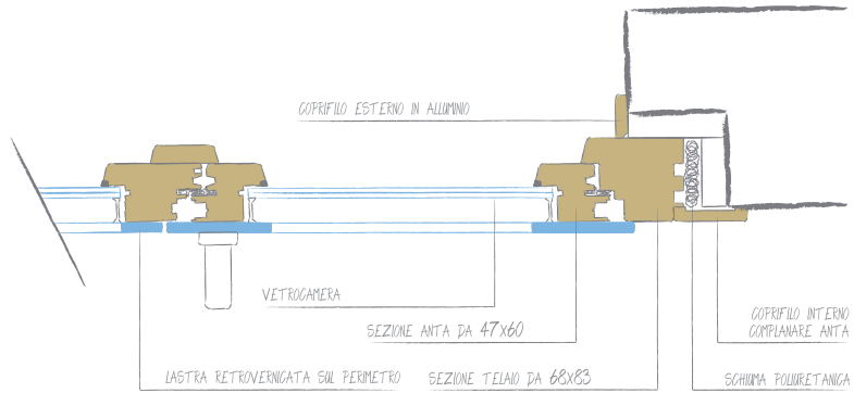
Sezione Orizzontale
