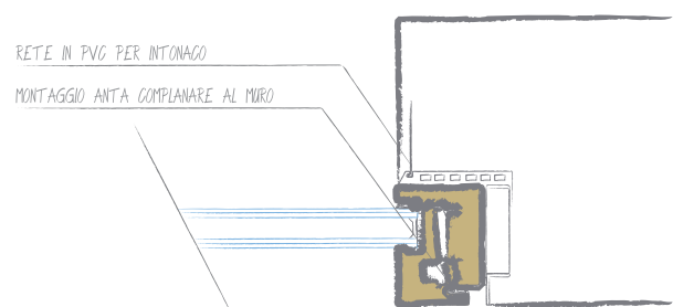
Sezione Orizzontale
