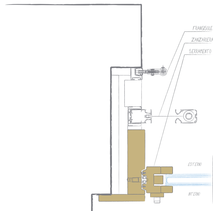
Sezione Orizzontale
