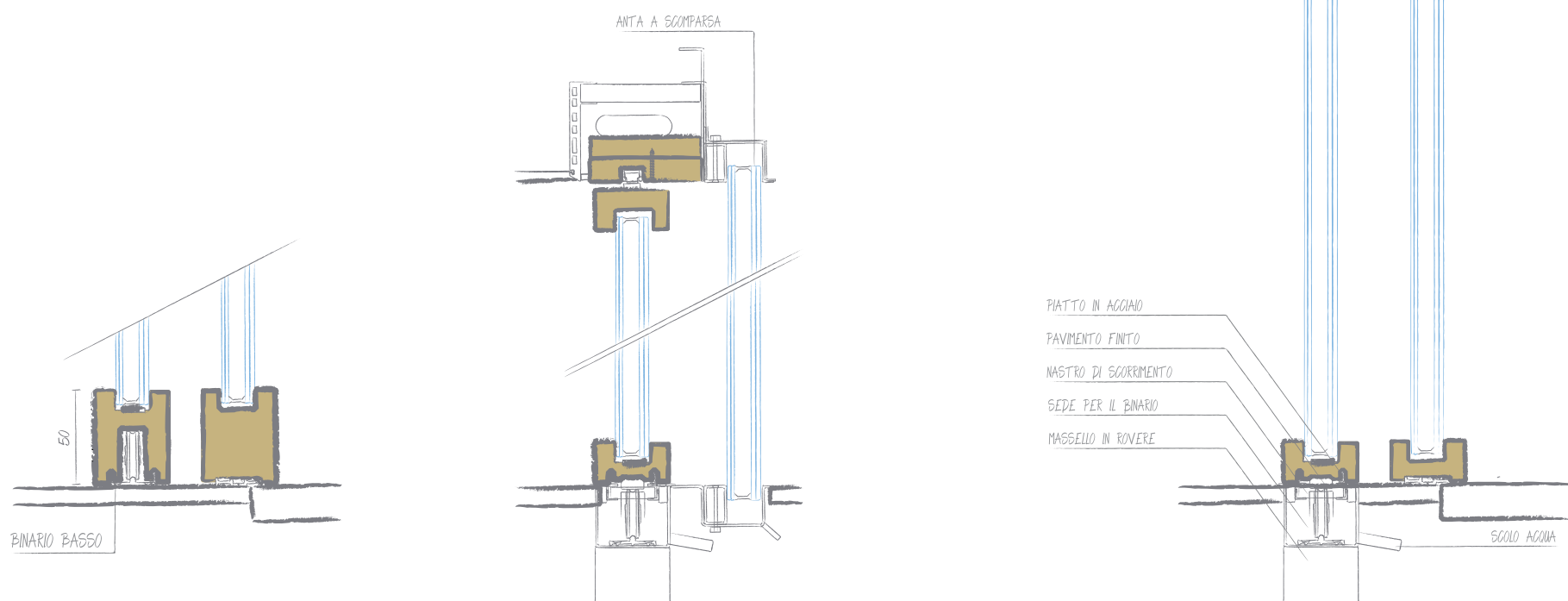
Sezione Verticale
