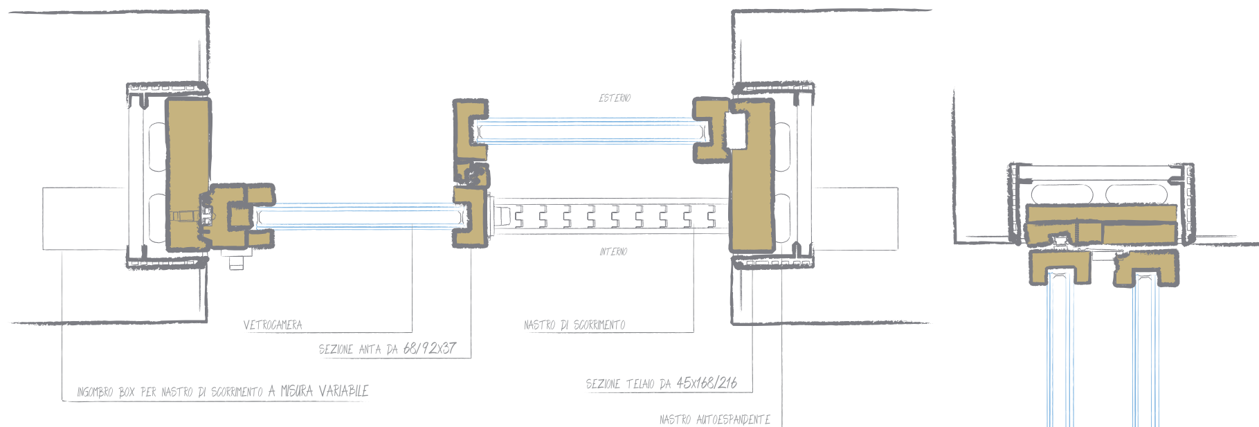
Sezione Orizzontale
