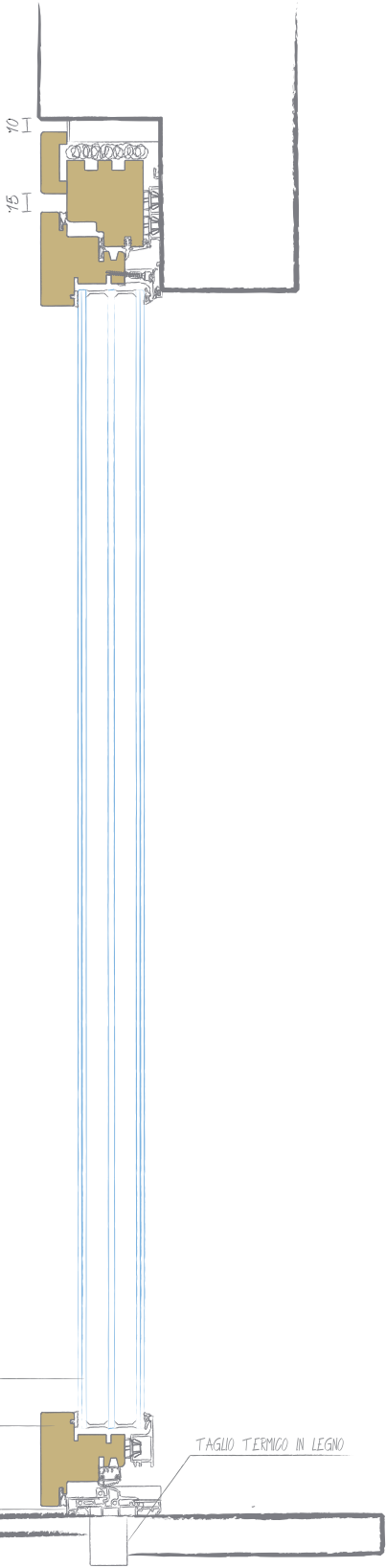
Sezione Verticale
