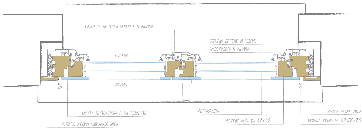
Sezione Orizzontale
