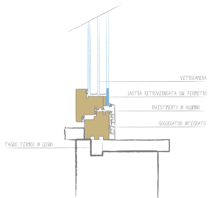
Sezione Verticale
