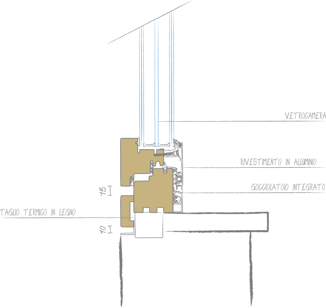
Sezione Verticale
