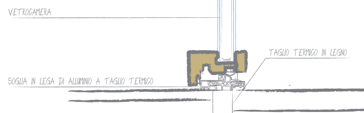
Sezione Verticale
