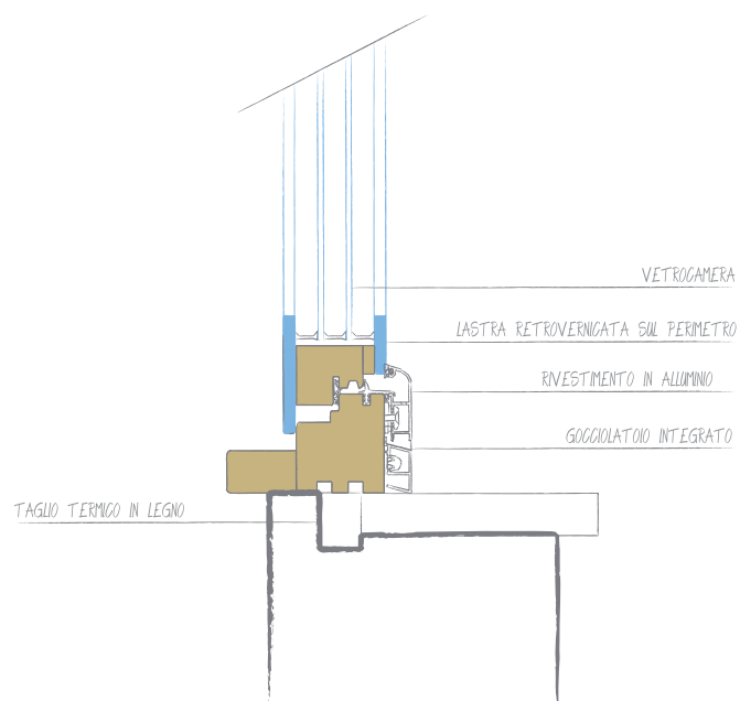
Sezione Verticale
