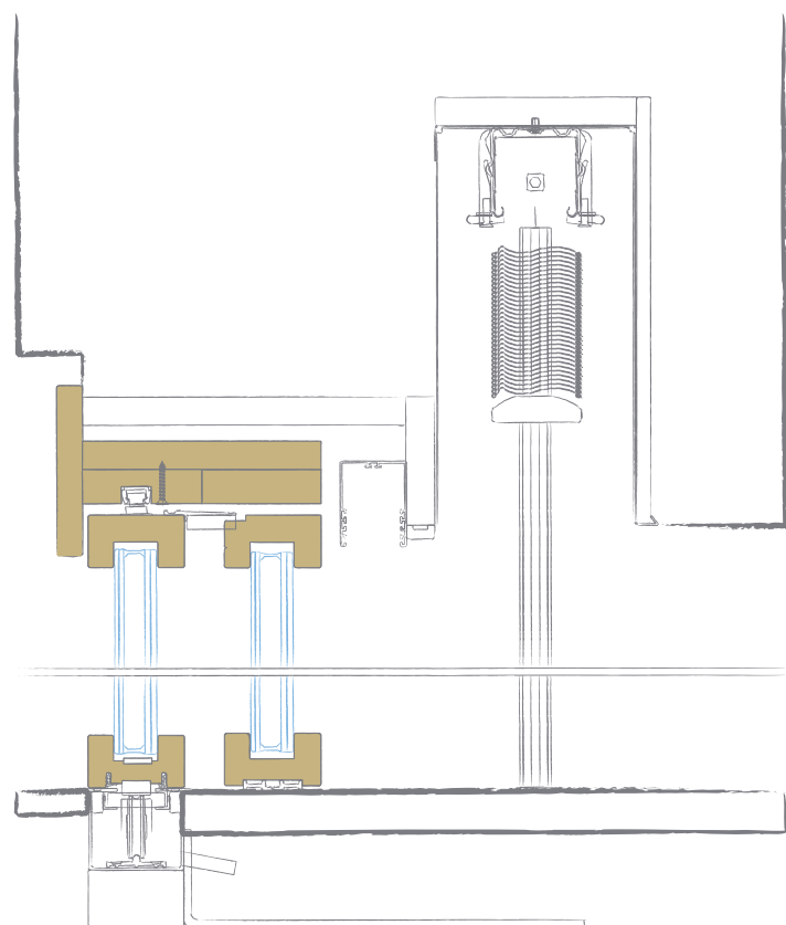
Sezione Verticale
