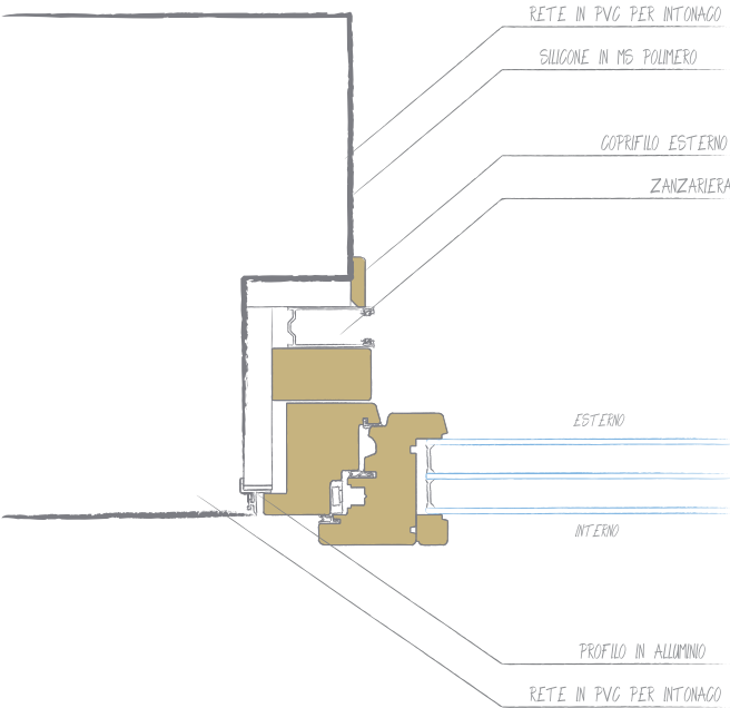
Sezione Orizzontale
