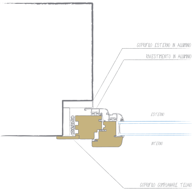
Sezione Orizzontale
