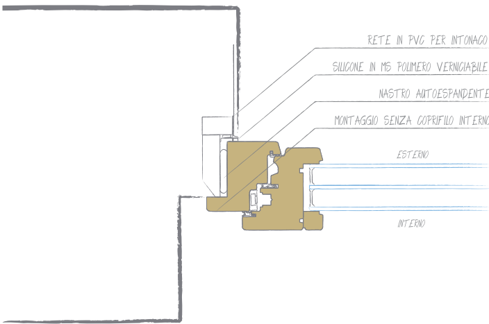
Sezione Orizzontale
