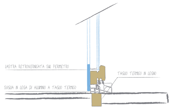
Sezione Verticale
