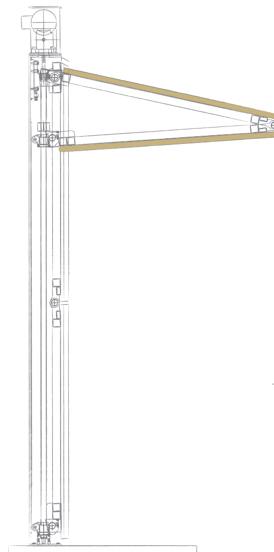
Sezione Verticale
