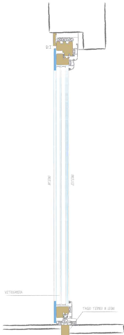
Sezione Verticale
