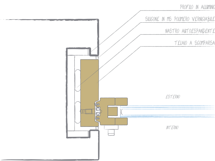
Sezione Orizzontale
