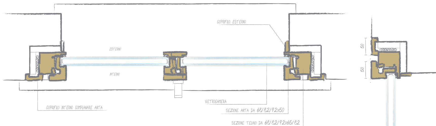
Sezione Orizzontale
