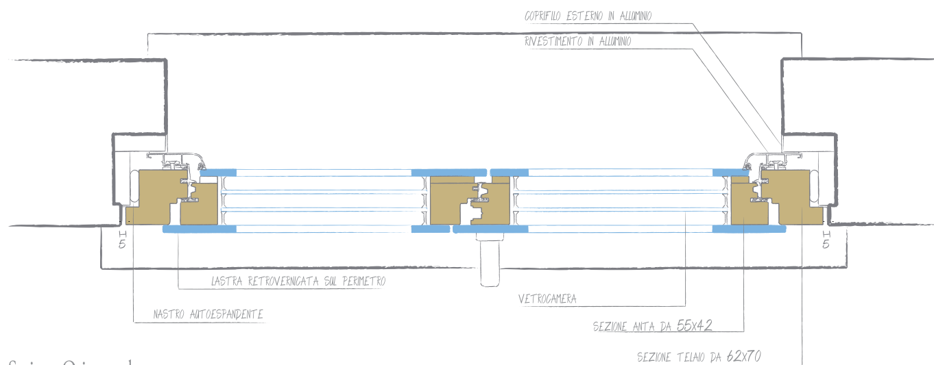
Sezione Orizzontale
