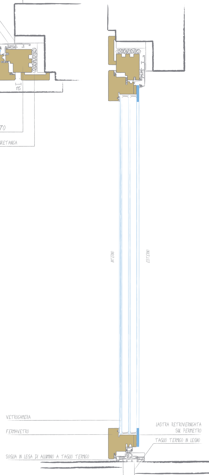
Sezione Verticale
