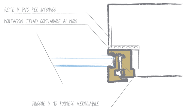
Sezione Orizzontale
