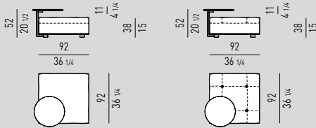
VERSIONE CON TAVOLINO | VERSION WITH SIDE TABLE
