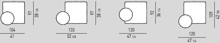
INGOMBRO POUF CON TAVOLINO | OTTOMAN WITH SIDE TABLE OVERALL DIMENSIONS
