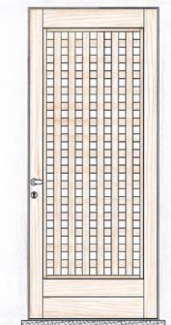
- PROSPETTO VISTA ESTERNA rif.1 - scala 1:10 - sol.D (con carabottino)
