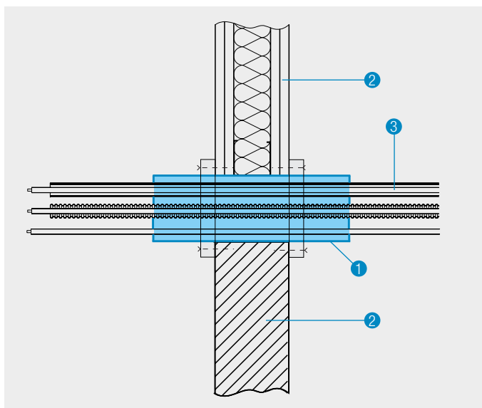
Particolare A - Sigillatura di cavi in pareti flessibili e rigide
