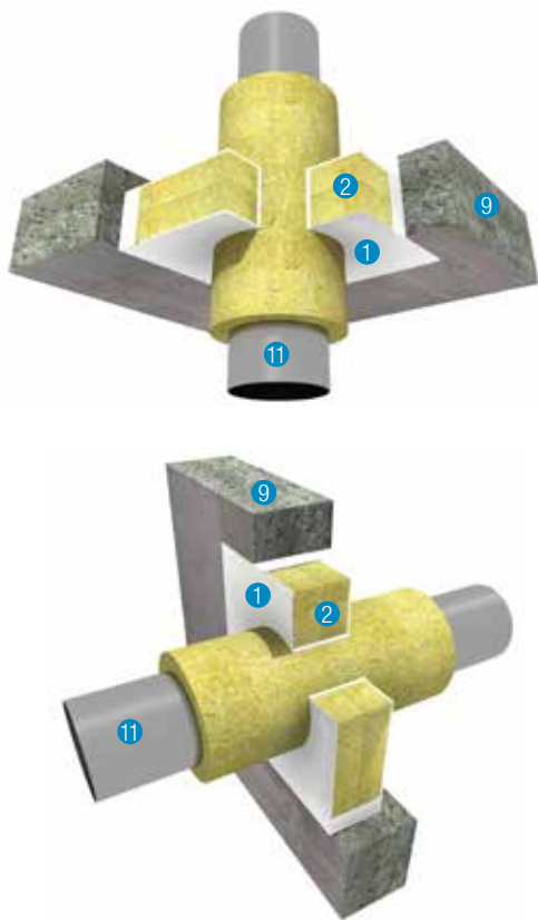
Particolare H - Sigillatura di tubo metallico in parete flessibile e parete rigida, Caso LS = locale sostenuto
