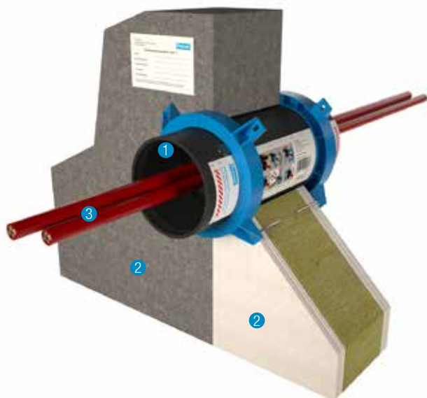
Particolare A - Sigillatura di cavi in pareti flessibili e rigide
