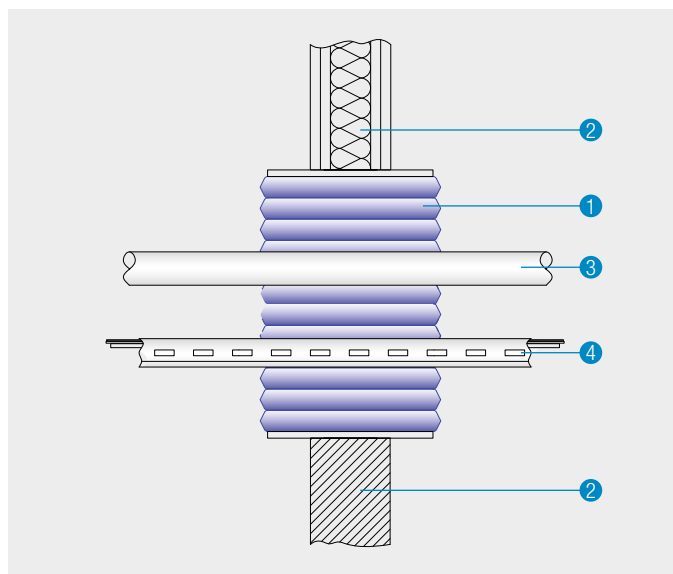
Particolare A - Sigillatura di tubazioni e impianti elettrici con PROMASTOP®-S/L in parete flessibile e parete rigida
