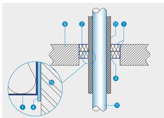
Particolare Y - Tubi metallici con isolante combustibile
