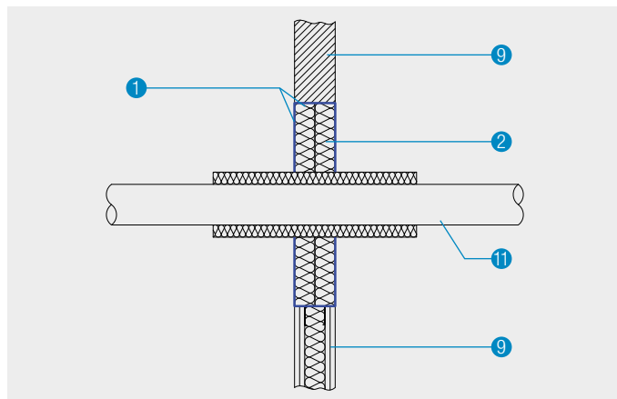
Particolare I - Sigillatura di tubo metallico in parete flessibile e parete rigida, Caso CS = continuo sostenuto
