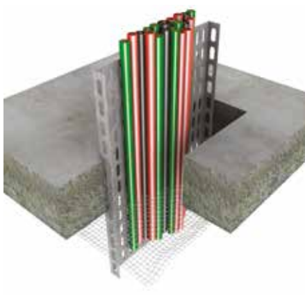
2. Solo per le applicazioni su supporti orizzontali: fissare una struttura di sostegno (per es. una rete in acciaio) all'intradosso del solaio
