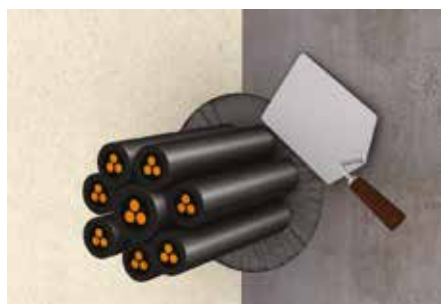
4. Stendere la superficie del sigillante prima della formazione della pellicola con un pennello o una spatola inumiditi con acqua
