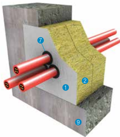
Particolare F - Sigillatura di cavi in parete flessibile e parete rigida
