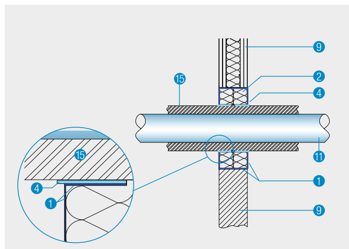
Particolare Z - Tubi metallici con isolante combustibile
