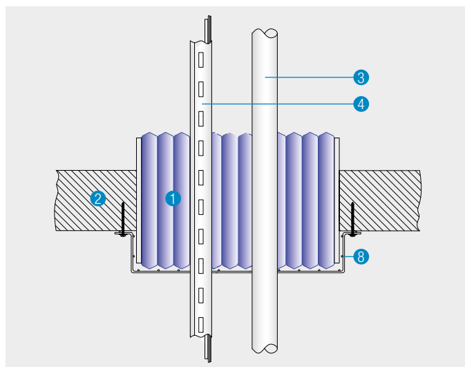
Particolare B - Sigillatura di tubazioni e impianti elettrici con PROMASTOP®-S/L in solaio rigido
