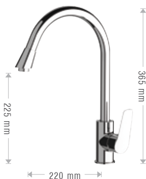
506/ES ESSENZA Miscelatore monocomando lavello bocca girevole. Single-lever sink mixer with swivel spout.
