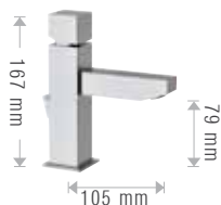
393/CB Miscelatore monocomando lavabo. Single lever basin mixer.
