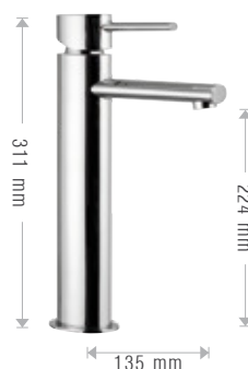
397/NU Miscelatore monocomando lavabo alto, senza scarico. Single lever basin mixer high neck without pop-up waste.
