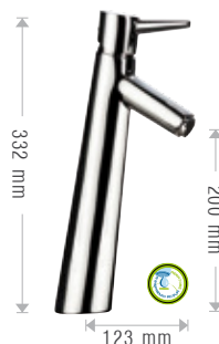
397/SN Miscelatore monocomando lavabo alto, senza scarico. Single lever basin mixer high neck, without waste.
