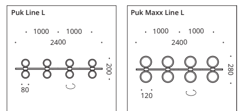
Kabellänge für Abhängung 2.000 mm (kürzbar) Cable length for suspension 2.000 mm (can be shortened)
