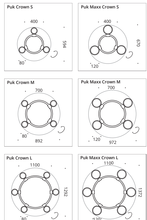
Kabellänge für Abhängung 3.000 mm (kürzbar) Cable length for suspension 3.000 mm (can be shortened)
