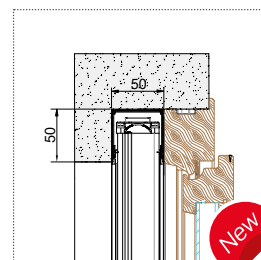
■ BORA INCAS MIDI DOPPIA 35/35
