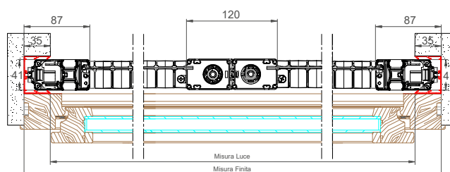
Apertura bilaterale
