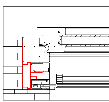
SEZIONE ORIZZONTALE
