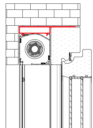
SEZIONE VERTICALE
