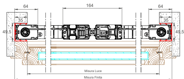
Chiusura centrale
