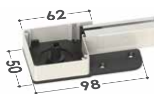
■ Cassonetto da 50 Testate inferiori
