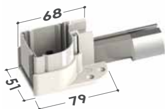
■ Cassonetto da 45
