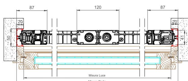
Apertura bilaterale
