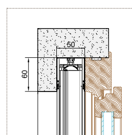
Apertura bilaterale
