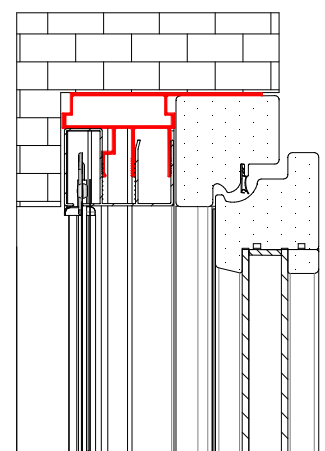
SEZIONE VERTICALE
