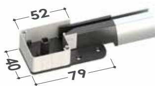
■ Cassonetto da 40 Testate inferiori
