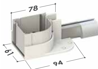
■ Cassonetto da 55
