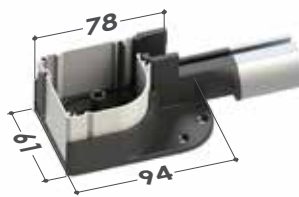
■ Cassonetto da 55 Testate inferiori
