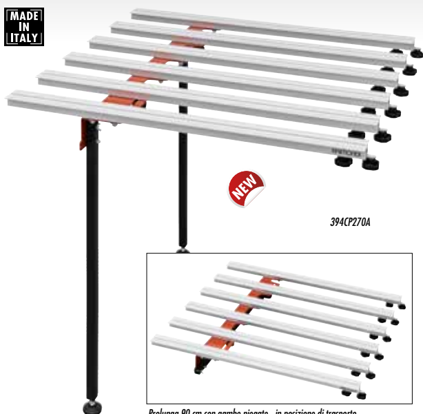
Prolunga 90 cm con gambe piegate - in posizione di trasporto
