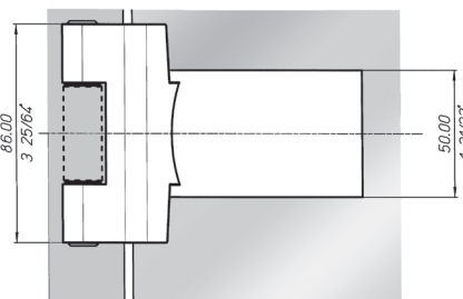
Perno doppio Double pin
