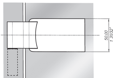
Perno singolo Single pin
