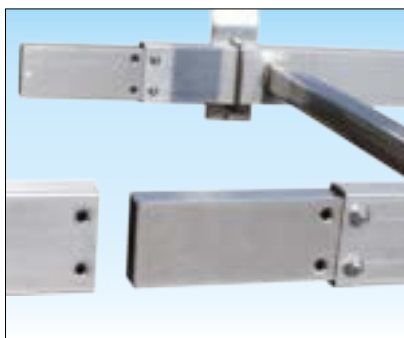
Spinotti di giunzione scala realizzati in robusto profilo rettangolo di alluminio !
