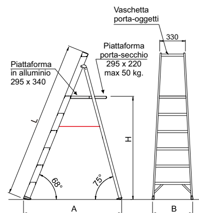
Grande piattaforma in robusto profilo d'alluminio dotata di ripiano PORTA-SECCHIO con portata 50kg.
