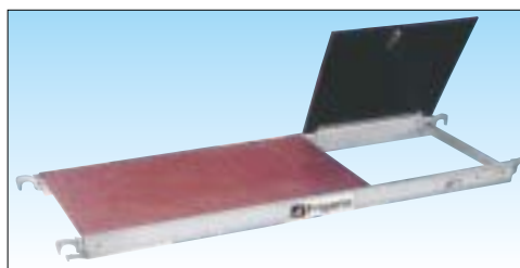
botola di passaggio cm 45 x 50 provvista di grilletto di bloccaggio automatico
