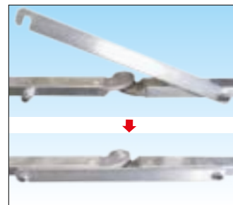
Sicurezza anti-chiusura del telaio ad aggancio rapido
