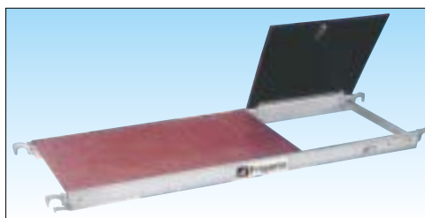
In foto struttura portante articolo ALP BASA20 con sbalzo ALP BASB20
