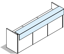
Reception W 107,6 / 207,6 / 307,6 D 84 – H 113,2
