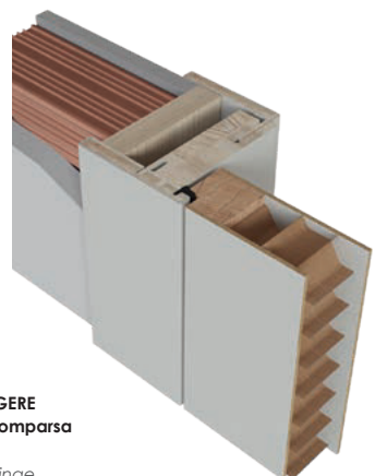
TELAIO STANDARD 1 con cerniera a scomparsa Special frame with concealed hinge
