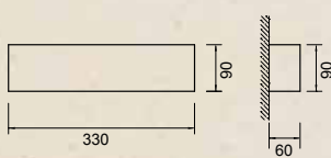
DIVETRO 33 Led 9W – 230Vac – 3000K CE Peso / Weight 0,75 kg
