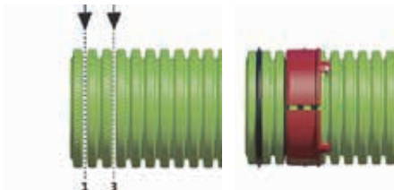
Posizionamento guarnizione di tenuta ed anello antisifilamento
