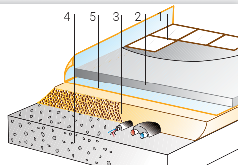
Sottofondi bistrato.
