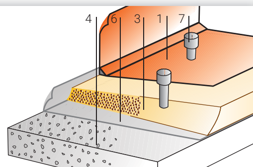
Coperture piane.
