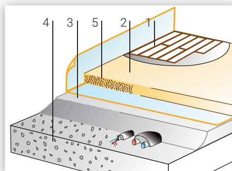
Sottofondi pluristrato.
