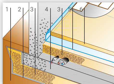
Vespaio isolato.
