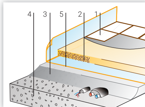
Sottofondi bistrato.
