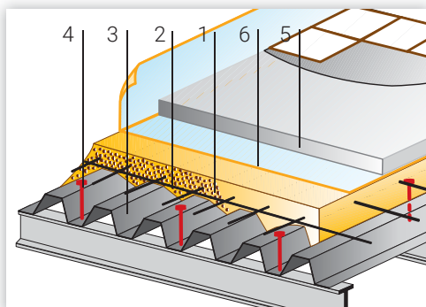
Solai metallici.
