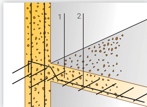
Getti strutturali.
