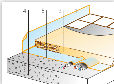
Sottofondi monostrato.
