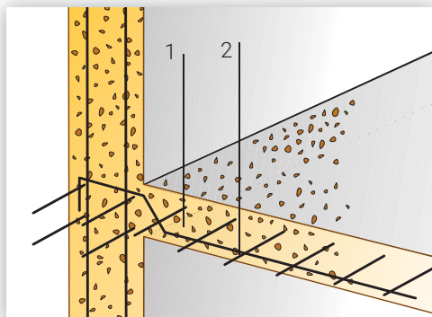
Getti strutturali.
