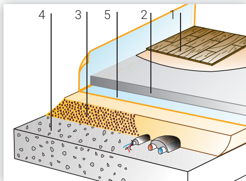
Sottofondi pluristrato.
