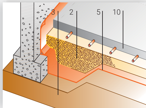
Isolamenti controterra.
