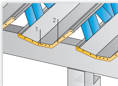
Strutture prefabbricate.
