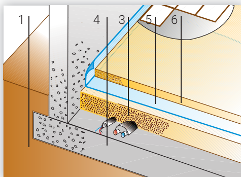
Sottofondo isolato.
