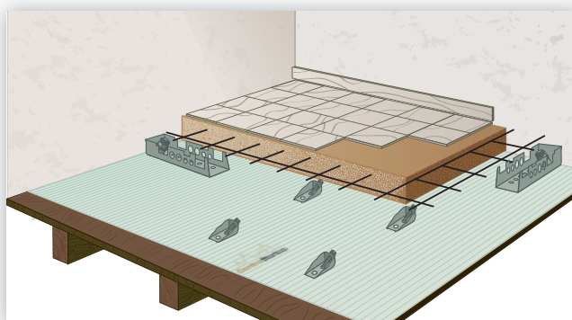
Collegamento solaio-pareti.
