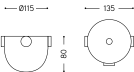
R4-3 Rosone decentramento con tre uscite Shifted light point with three outputs
