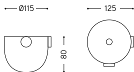
R4-90° Rosone con due uscite a 90° Ceiling rose with two 90° outputs
