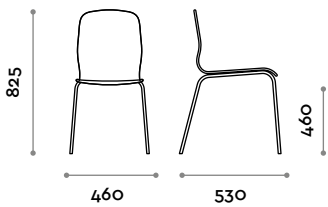
Dimensioni L 460 mm / P 530 mm / H 825 mm
