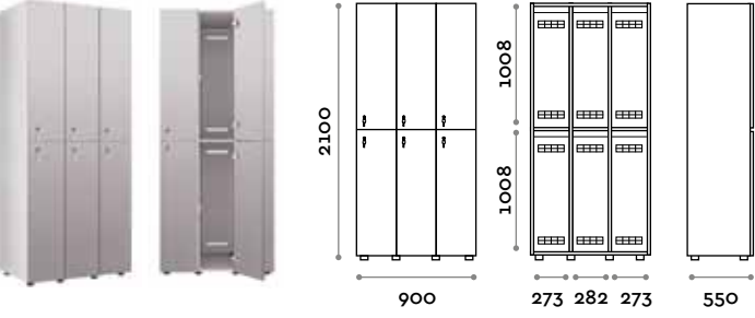
ANB90-19 Armadio triplo 6 ante
