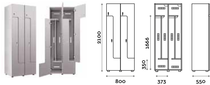
VANB34 Armadio singolo 1 ante per panca
