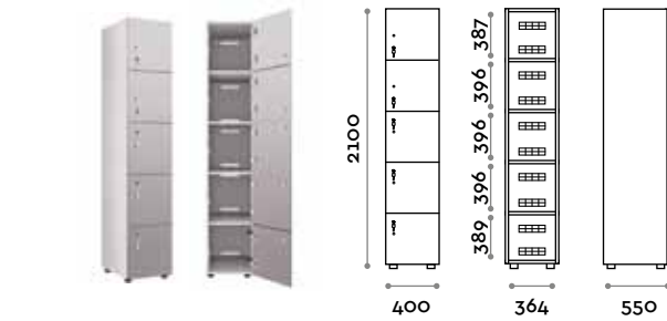
VANB426 Armadio doppio 6 ante con gancio
