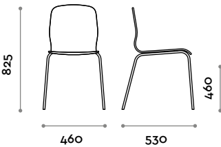
Dimensioni L 460 mm / P 530 mm / H 825 mm
