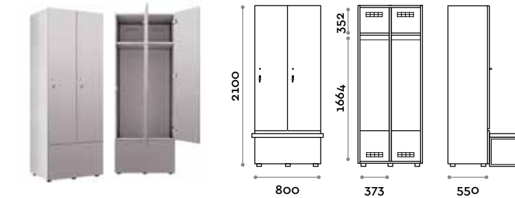
VANB35 Armadio singolo 2 ante per panca
