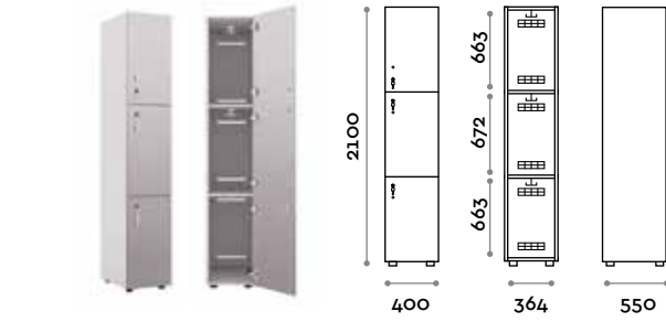
VANB324 Armadio singolo 4 ante
