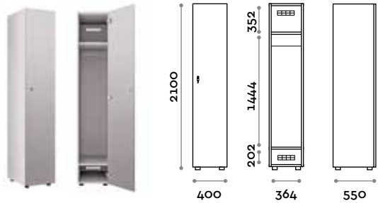
ANB41-19 Armadio doppio 2 ante
