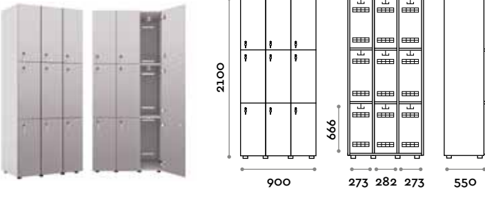
ANB93-19 Armadio triplo 9 ante con gancio
