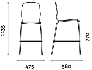
Dimensioni L 475 mm / P 580 mm / H 1135 mm
