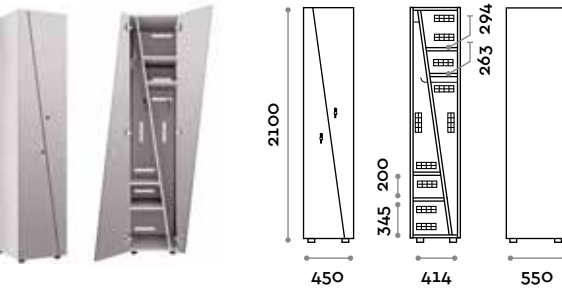
ATRO2-19 Armadio 2 ante trapezoidali
