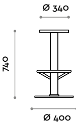
Dimensioni Ø 400 mm / H 820 mm
