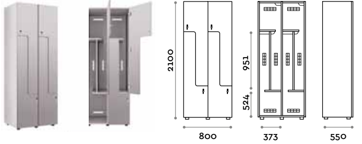
ANB49-19 Armadio doppio 4 ante a "L"
