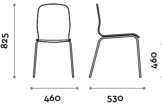
Dimensioni L 460 mm / P 530 mm / H 825 mm
