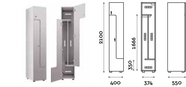
VANB48 Armadio doppio 4 ante a "L"
