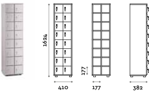
APV16 Portavalori 16 porte
