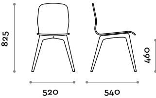
Dimensioni L 520 mm / P 540 mm / H 825 mm
