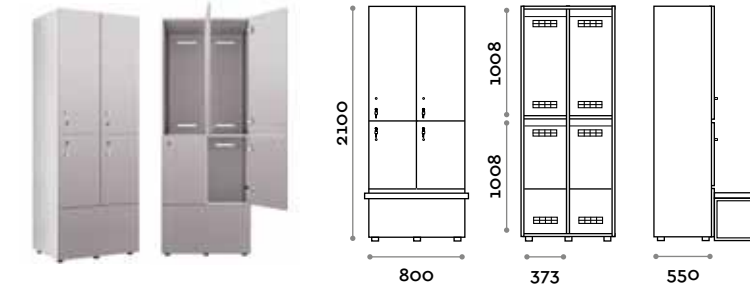
VANB45 Armadio doppio 4 ante per panca
