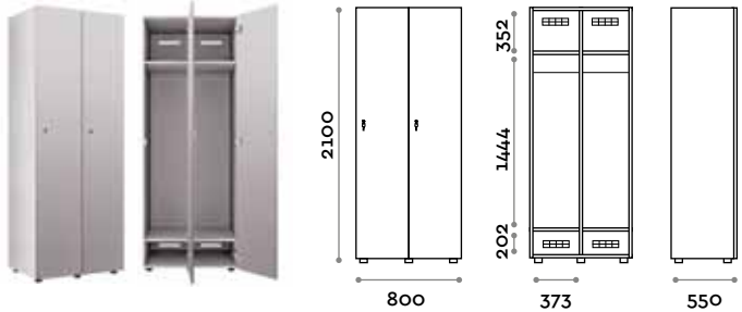
ANB32-19 Armadio singolo 2 ante
