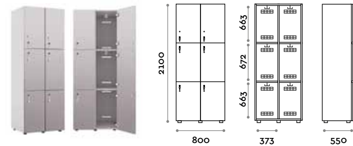
VANB428 Armadio doppio 8 ante
