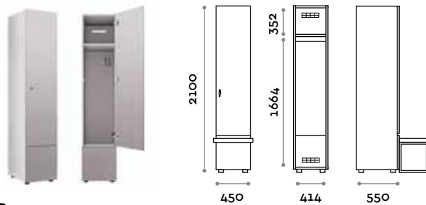
ANB12-19 Armadio 2 ante per panca
