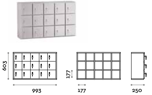
APVCHNW Pensile ricarica smartphone
