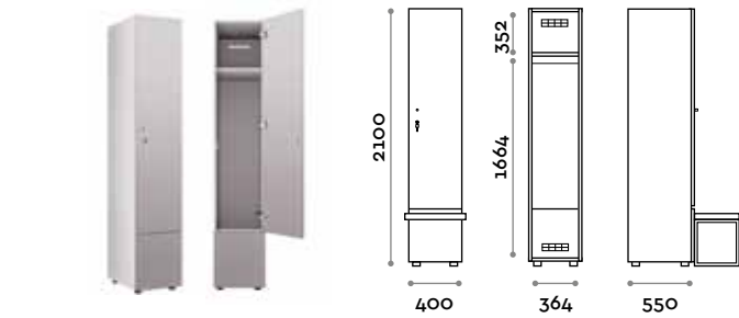
VANB44 Armadio doppio 2 ante per panca
