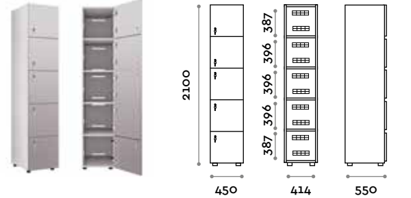
ANB05-19 Armadio 5 ante
