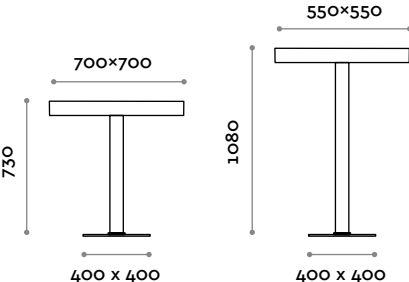
QUADRA C Dimensioni base 400x400 mm / top 700x700 mm / H 730 mm
