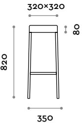
Dimensioni L 350 mm / P 350 mm / H 820 mm
