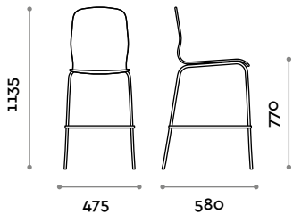
Dimensioni L 475 mm / P 580 mm / H 1135 mm
