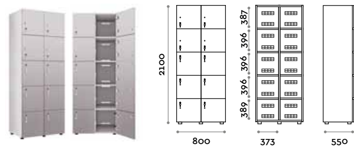
VANB4210 Armadio doppio 10 ante
