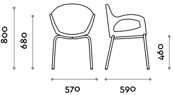
Dimensioni L 570 mm / P 590 mm / H 800 mm
