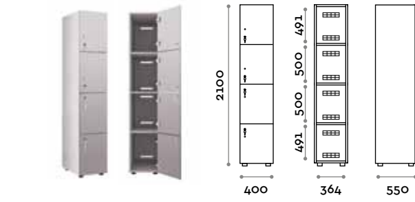
VANB325 Armadio singolo 5 ante
