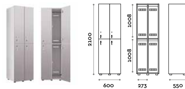
VANB60 Armadio doppio 4 ante
