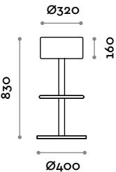
Dimensioni Ø 400 mm / H 825 mm
