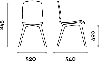
Dimensioni L 520 mm / P 540 mm / H 845 mm
