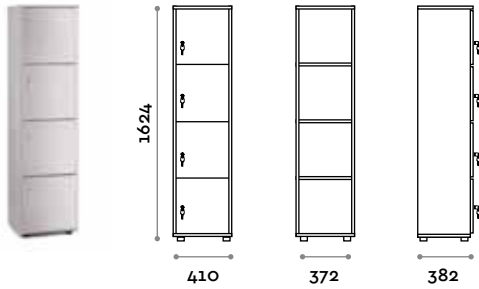
APV10 Portavalori 10 porte
