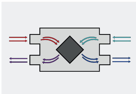
Fig. 2.6 Gli scambiatori di calore statici vengono attraversati dai due flussi dell'aria viziata e di quella fresca in modo da trasferire il calore senza mai miscelarsi fra loro.
