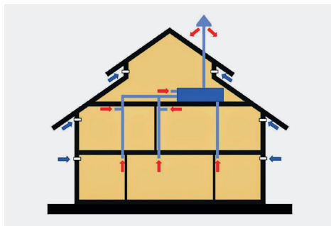
Fig. 2.1 Nei sistemi monoflusso l'unità di ventilazione estrae l'aria dai locali meno nobili. L'immissione di aria fresca e pulita avviene dai locali più nobili.
