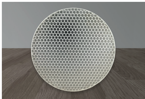
Fig. 4.1 Recupерatore rigenerativo in ceramica porosa, che negli apparati a singolo flusso ciclico funge da massa di accumulo del calore. Durante l'estrazione dell'aria la ceramica accumula una parte del calore contenuto nell'aria in uscita e durante la successiva fase di immissione il calore viene restituito. Come è logico aspettarsi, i massimi valori di scambio termico avvengono durante i primissimi istanti successivi all'inversione del ciclo di funzionamento, poiché in questa fase le differenze di temperatura fra l'aria e la massa ceramica sono più marcate.
