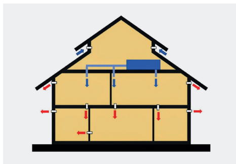
Fig. 2.3 Sistema monoflusso a pressione positiva.
