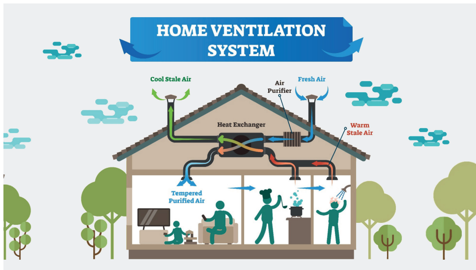
Fig. 2.4 Nei sistemi di ventilazione meccanica a doppio flusso le portate di mandata e di ripresa sono identiche e non si verificano depressioni nei locali.
