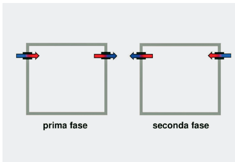
Fig. 4.3 Per garantire il loro corretto funzionamento, i sistemi a singolo flusso ciclico devono sempre essere installati in coppia, così che quando uno estrae l'altro immette e viceversa. Durante la prima fase, l'apparato di sinistra dell'immagine immette l'aria fredda nel locale riscaldandola e quello di destra contemporaneamente la estrae cedendo calore alla massa di ceramica. Nella seconda fase il funzionamento si inverte, l'apparato di sinistra estrae l'aria dal locale scaldando la massa ceramica e quello di destra immette l'aria dall'esterno recuperando una parte del calore precedentemente accumulato.
