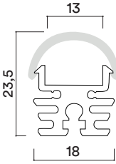
Dimensiones en mm Dimensions in mm
