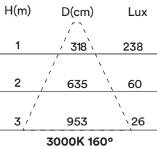
Curva fotométrica - Photometric curve
