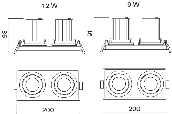
Dimensiones en mm - Dimensions in mm
