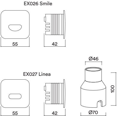
Dimensiones en mm - Dimensions in mm
