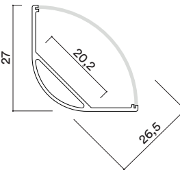
Dimensiones en mm Dimensions in mm
