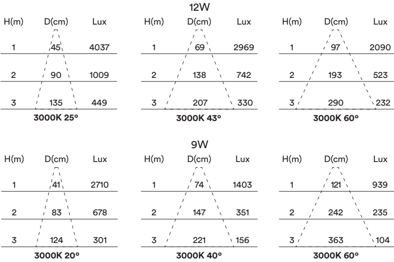
Curva fotométrica - Photometric curve
