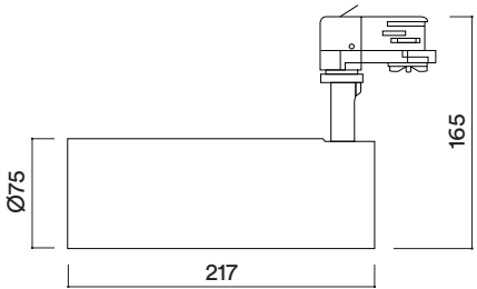
Dimensiones en mm - Dimensions in mm
