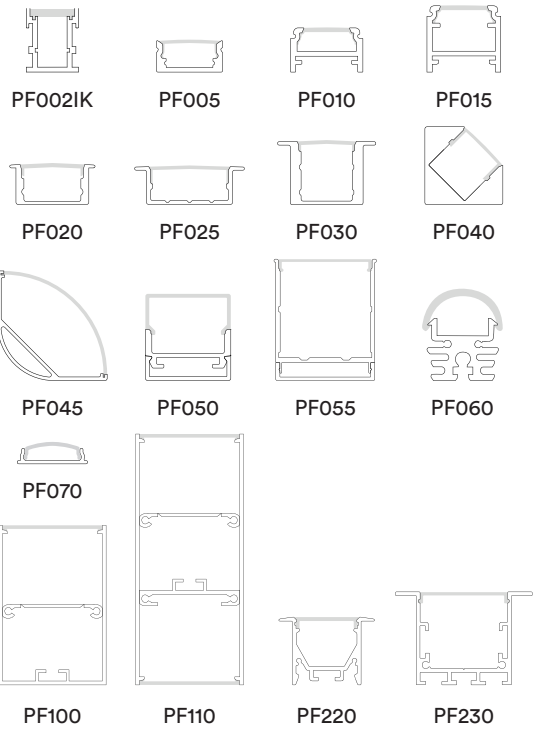
Dimensiones en mm - Dimensions in mm
