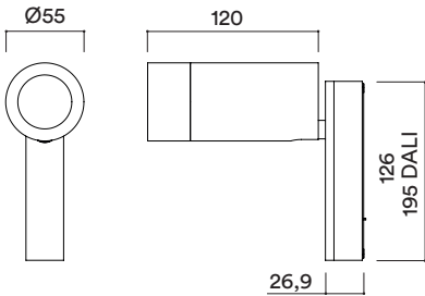
Dimensiones en mm - Dimensions in mm
