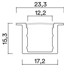
Dimensiones en mm Dimensions in mm
