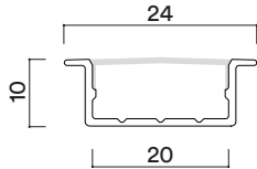
Dimensiones en mm Dimensions in mm
