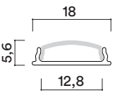
Dimensiones en mm Dimensions in mm
