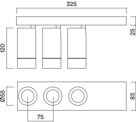
Dimensiones en mm - Dimensions in mm
