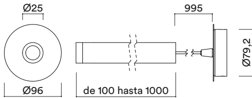
Dimensiones en mm - Dimensions in mm
