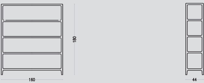
Bellagio bookcase Art 6201/F Libero Rutilo
