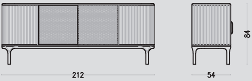
Fantesca sideboard Art 1703 Maurizio Duranti
