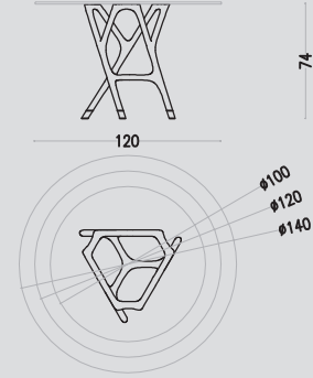
Joyce Round Table Art 5705/F Libero Rutilo
