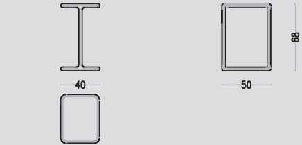
Bellagio Small Table Art 5627/F Libero Rutilo
