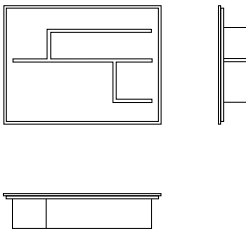
Art. RC 143 Pannello plasma con mensola Plasma panel with shelves Плазменная панель с полками L. 160 H. 120 P. 27
