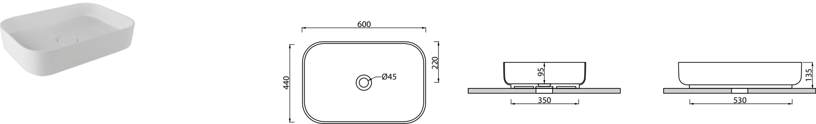
_LAVABO QUBE 9 Art. LVQ9 Lavabo rettangolare da appoggio 60x44 cm senza troppopieno Laid on rectangular washbasin 60x44 cm without overflow
