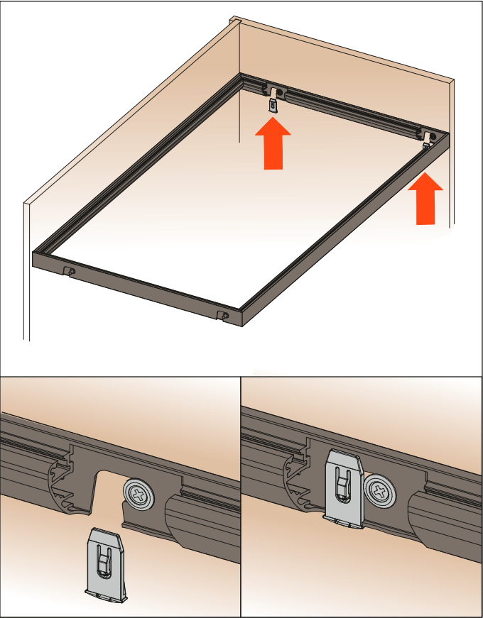
4. Inserire la clip di bloccaggio
