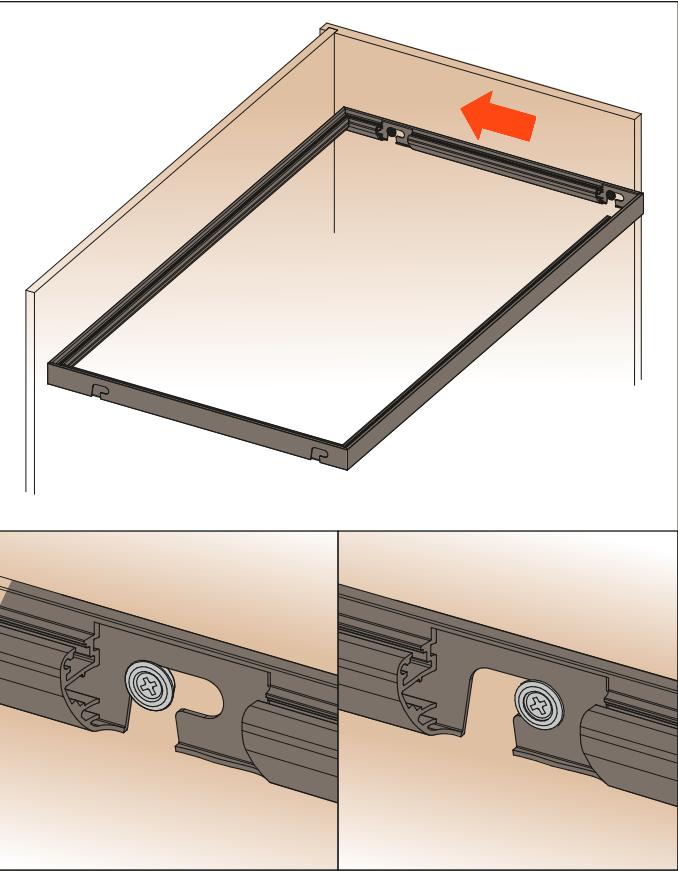
3. Far scorrere il ripiano per bloccarlo al supporto
