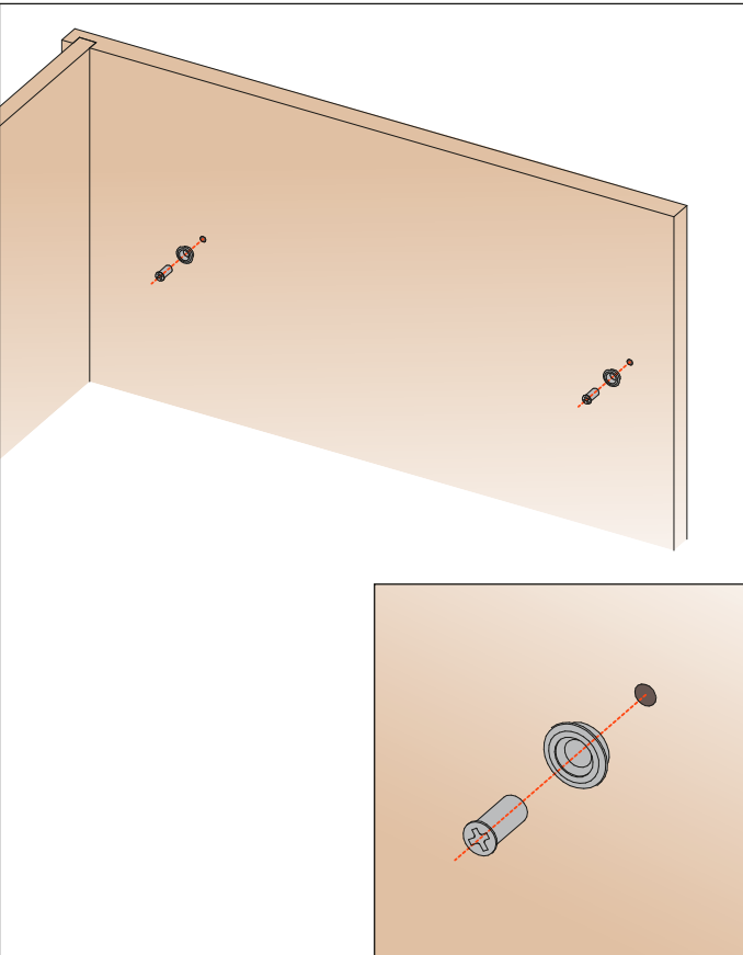
1. Avvitare i supporti al fianco del mobile
