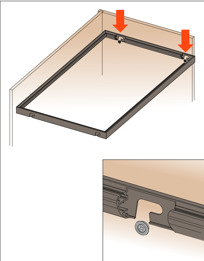
2. Inserire il ripiano sui supporti
