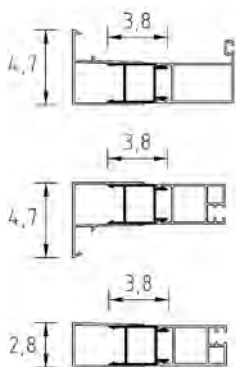
PER SERIE EUROPA - EUROPA SP - CEE ART - AMERICA QUATTRO Profilo di compensazione
