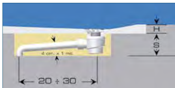
STONEFIT incassato a filo pavimento
