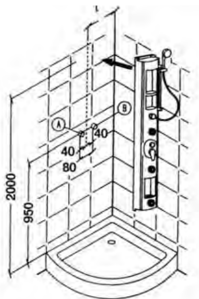
Montaggio a parete
