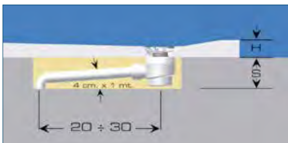
STONEFIT incassato in appoggio a pavimento
