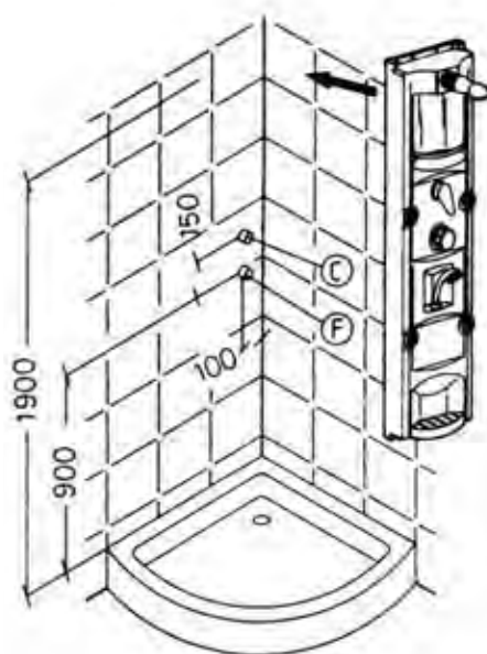
Montaggio ad angolo
