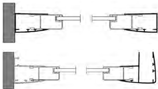
Corretta installazione del profilo ad angolo
