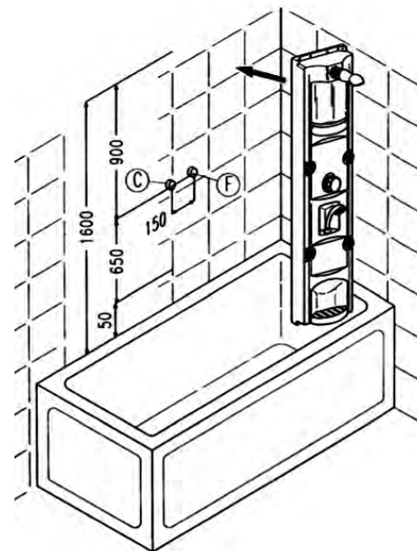
Montaggio per vasche da bagno
