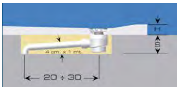
STONEFIT incassato in appoggio a pavimento
