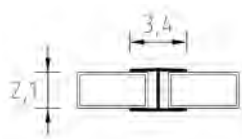
PER SERIE CON PANNELLI IN POLYSTYRENE Profilo di congiunzione
