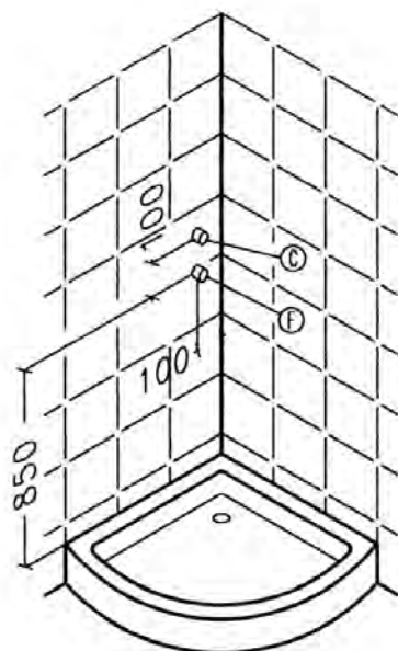
Solo montaggio ad angolo
