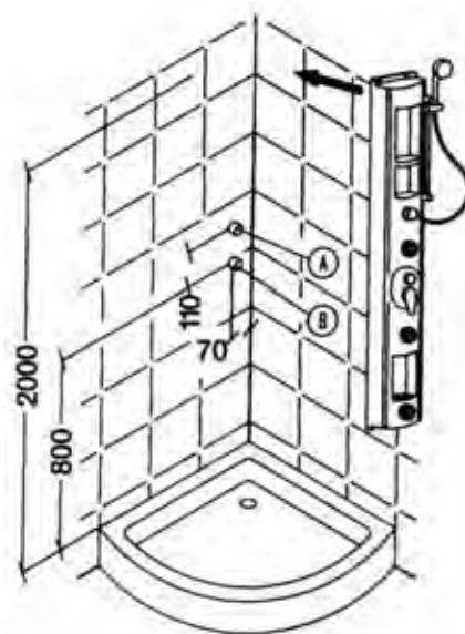
Montaggio ad angolo
