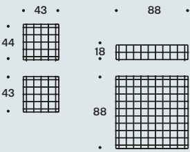
Tavolini / Low tables
