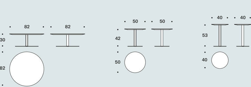
Tavolini / Low tables
