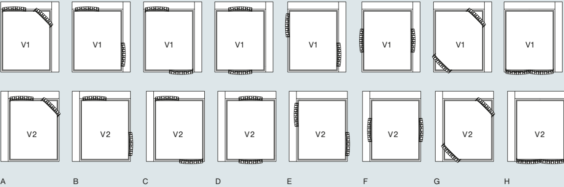
Esempi posizione pannelli testiera / Examples headboard panels position
