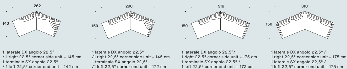
Esempi composizioni angolo 22,5° / Examples of 22,5° corner compositions
