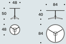
Tavolini tondi / Round low tables
