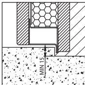
Battuta Floor Threshold Притвор MIN 15
