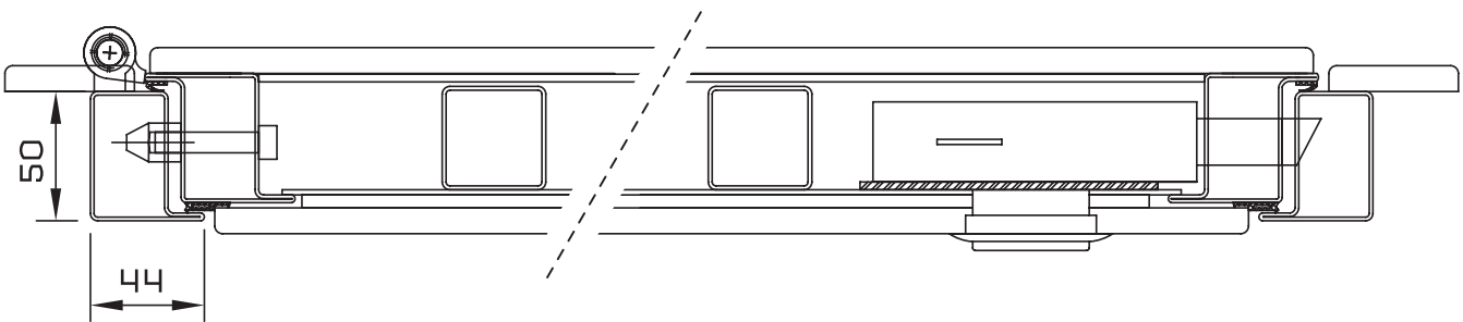
2 ANTE • 2 LEAVES • ДВУХСТВОРЧАТАЯ ДВЕРЬ
