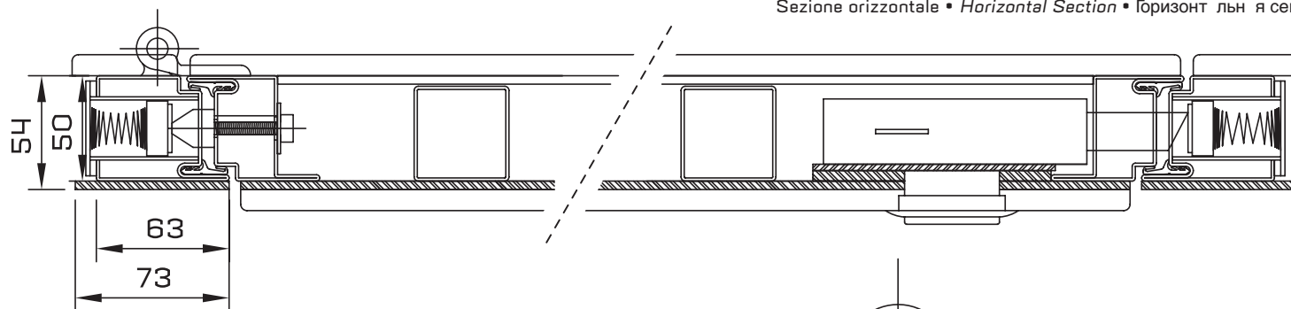
Sezione orizzontale • Horizontal Section • Горизонтальная секция
