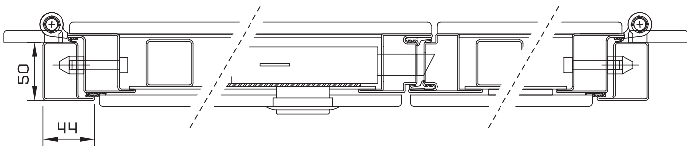
2 ANTE • 2 LEAVES • ДВУХСТВОРЧАТАЯ ДВЕРЬ
