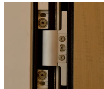
Cerniere invisibili • Hidden hinges • скрытые петли
