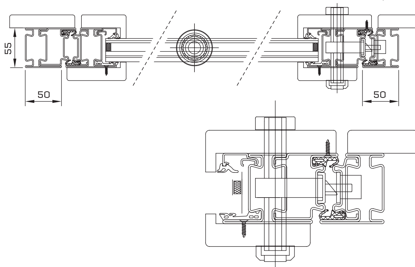
Sezione orizzontale • Horizontal Section • Горизонтальная секция
