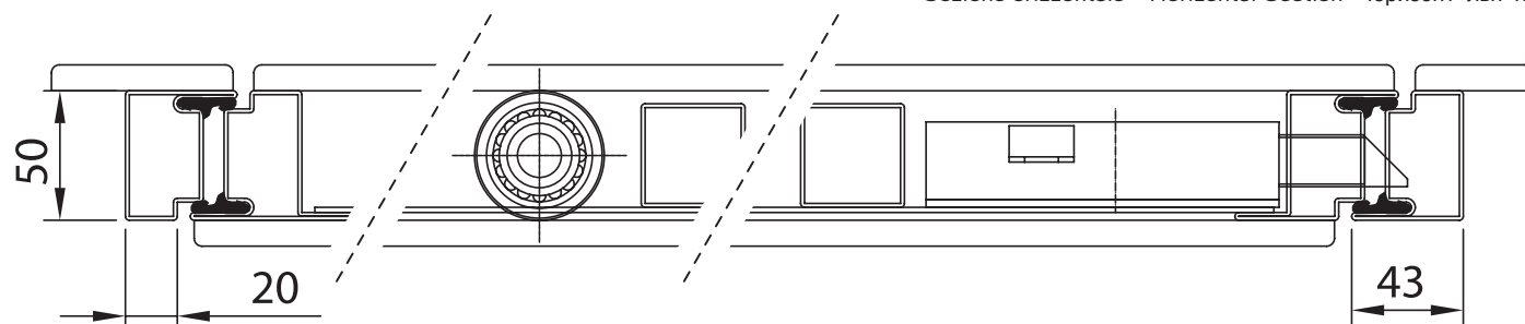
Sezione orizzontale • Horizontal Section • Горизонтальная секция
