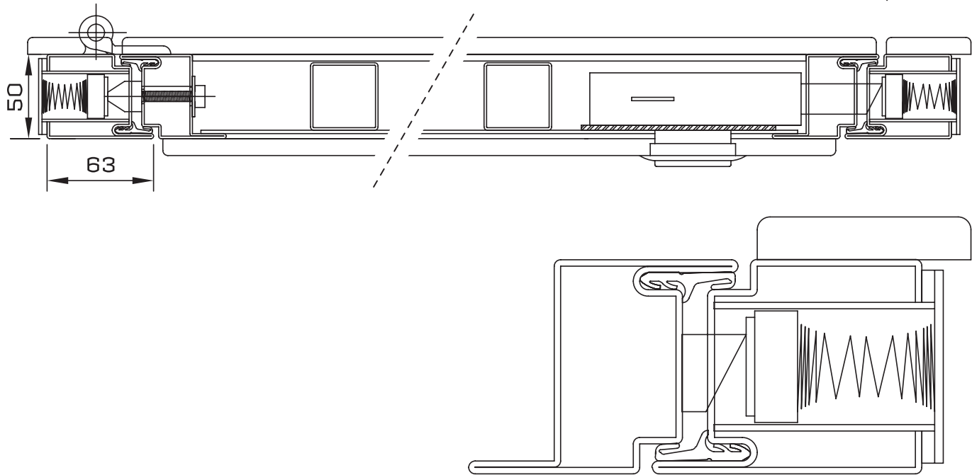
Sezione orizzontale • Horizontal Section • Горизонтальная секция
