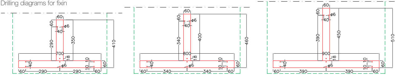
Schemi foratura per fissaggi Drilling diagrams for fixin
