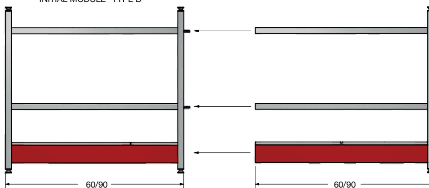
MODULO INIZIALE "TIPO B" INITIAL MODULE "TYPE B"
