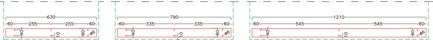
Schemi foratura per fissaggi Drilling diagrams for fixin
