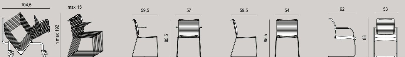
SEDUTA ATTESA CON E SENZA BRACCIOLI + CANTILEVER | WAITING CHAIR WITH AND WITHOUT ARMRESTS + CANTILEVER
