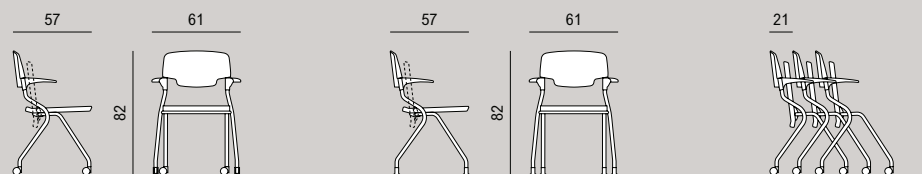
SEDUTA ATTESA IMBOTTITA CON BRACCIOLI | PADDED WAITING CHAIR WITH ARMRESTS
