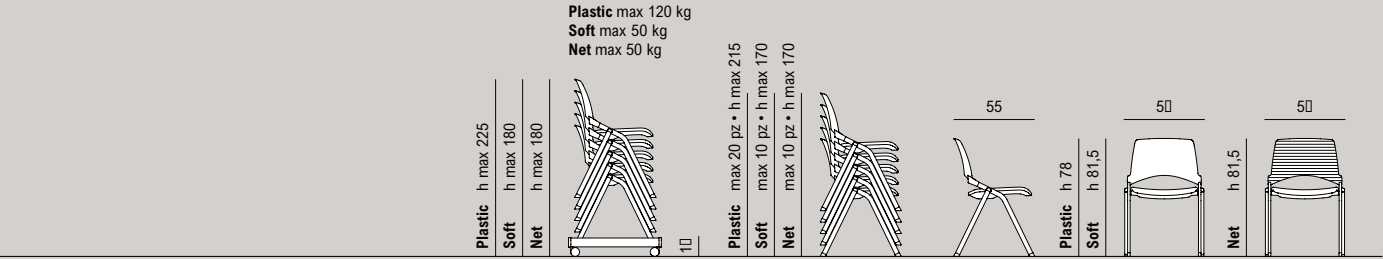
SEDUTA ATTESA | WAITING CHAIR
