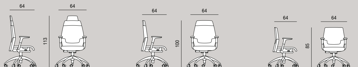
SEDUTA PRESIDENZIALE, DIREZIONALE E SEMIDIREZIONALE | HIGH EXECUTIVE, EXECUTIVE AND MANAGER CHAIR
