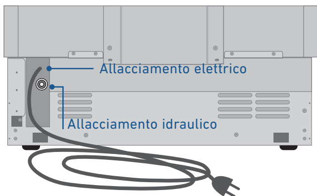
fig.1 Retro dell'apparecchiatura
