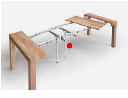
L'apertura avviene attraverso un cavalletto centrale in acciaio e guida in alluminio. The console table opens out thanks to a central steel stand and aluminium guide.
