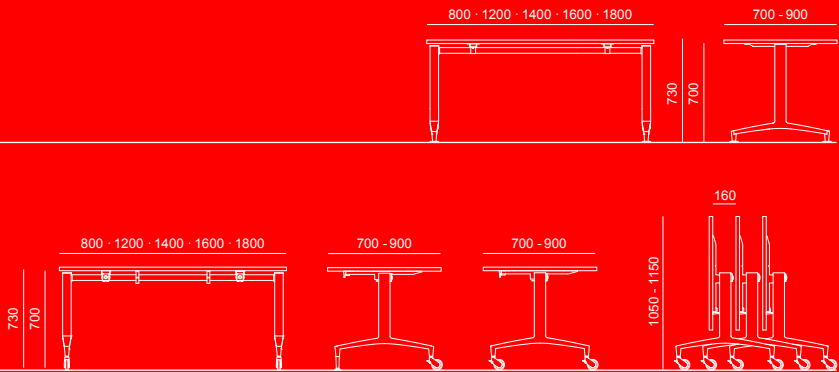
TAVOLO RIBALTABILE CON RUOTE E PIEDINI COMPENSATORI | FLIP TOP TABLE WITH CASTORS AND ADJUSTABLE GLIDES
