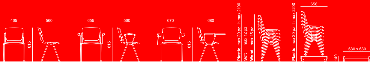
SEDIA CON E SENZA BRACCIOLI E SCRITTOIO | CHAIR WITH OR WITHOUT ARMS AND WRITING TABLET
