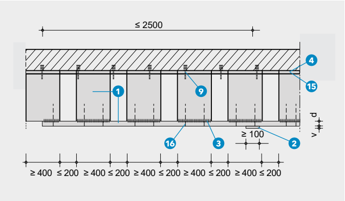
DETTAGLIO T – SEZIONE LONGITUDINALE
