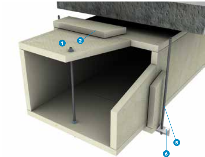
DETTAGLIO A - SEZIONE TRASVERSALE
