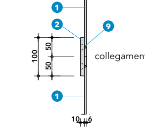
DETTAGLIO C.1
