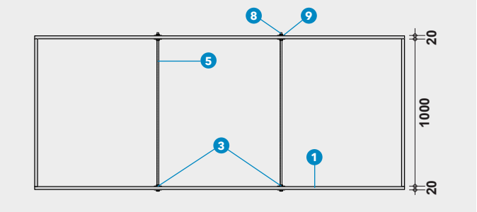
DETTAGLIO D - SEZIONE TRASVERSALE CONDOTTE GRANDI CON SOSPENSIONE
