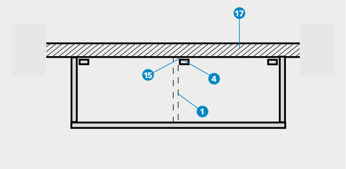
DETTAGLIO S – RINFORZO INTERNO - SEZIONE TRASVERSALE
