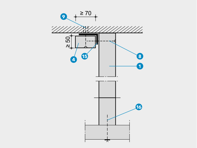
DETTAGLIO T – SEZIONE LONGITUDINALE
