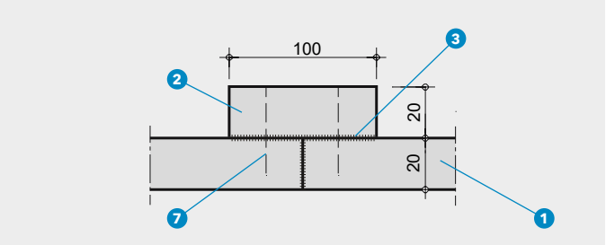
DETTAGLIO G - COLLEGAMENTO DI SPIGOLO
