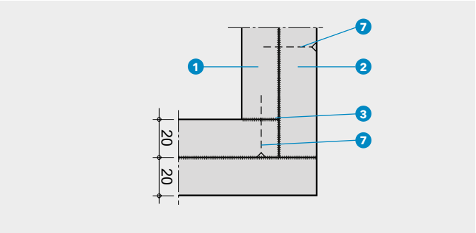
DETTAGLIO G - COLLEGAMENTO DI SPIGOLO
