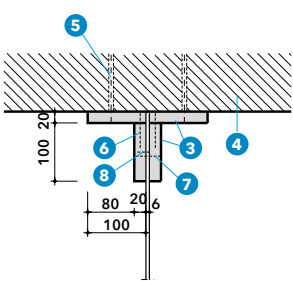
DETTAGLIO B.1
