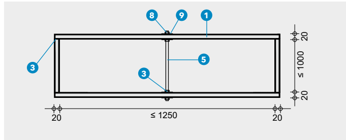
DETTAGLIO A - SEZIONE TRASVERSALE
