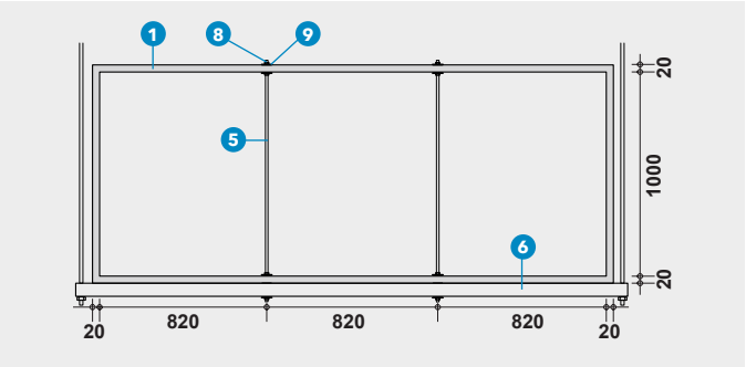
DETTAGLIO E - SISTEMA DI SOSPENSIONE
