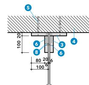
DETTAGLIO B.2 (ALTERNATIVA)
