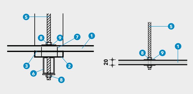
DETTAGLIO F - COLLEGAMENTO TR DUE SEZIONI
