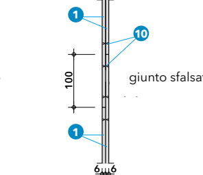
DETTAGLIO C.2 (ALTERNATIVA)
