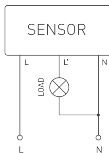
Рисунок 3. Схема подключения.
