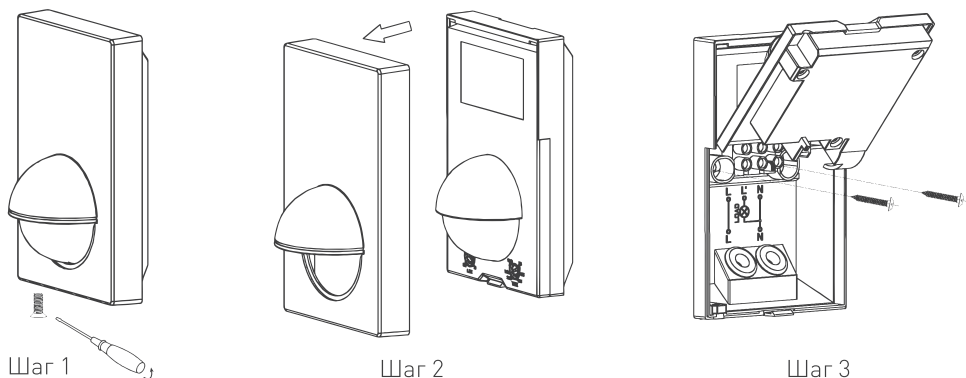
Рисунок 1. Этапы монтажа датчика.
