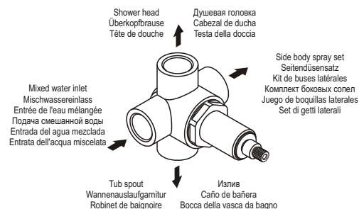
4-way valve • Vierwegeventil • Soupape à 4 voies 4-ходовой клапан • Válvula de 4 vías • Valvola a 4-vie
