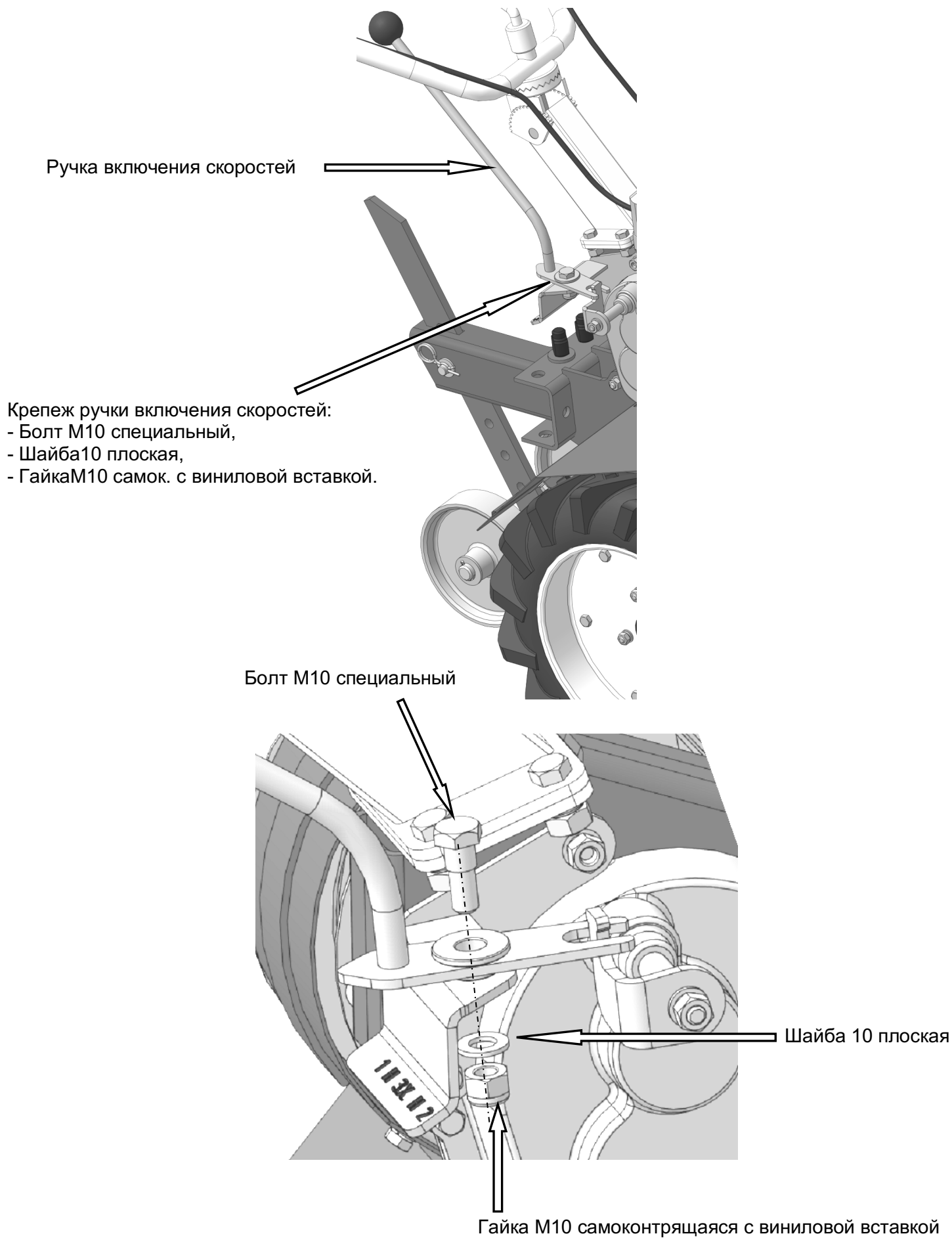
Рис.5. Схема сборки мотоблока с ручкой включения скоростей.
