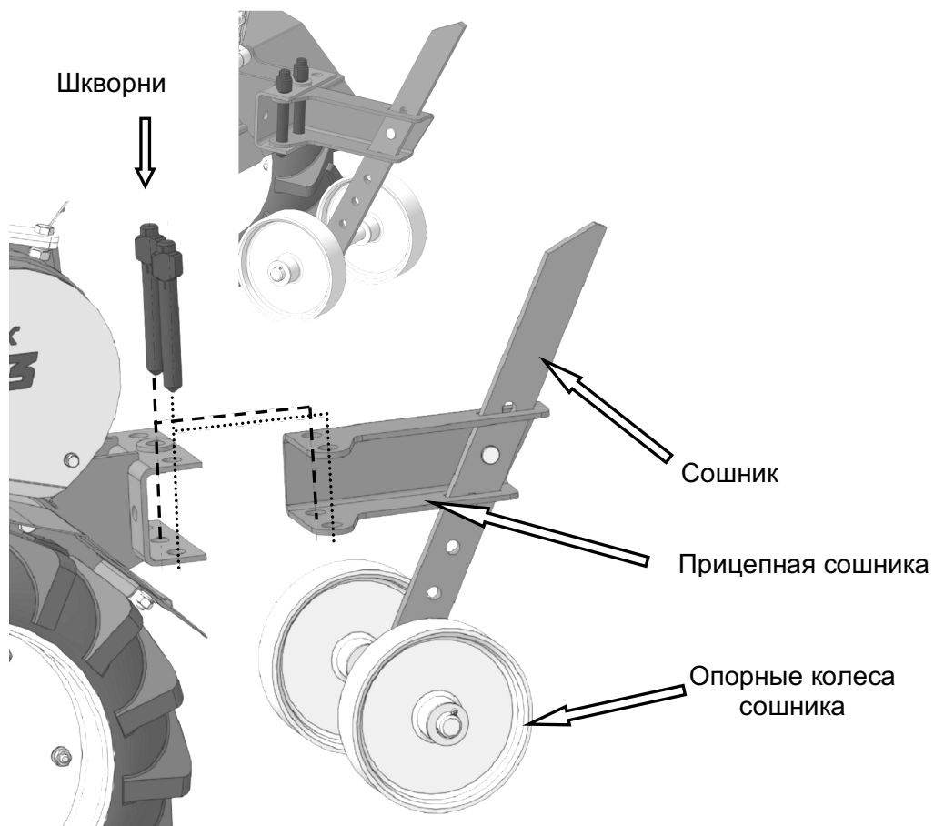
Рис.3. Схема сборки мотоблока с прицепной сошника и сошником.
