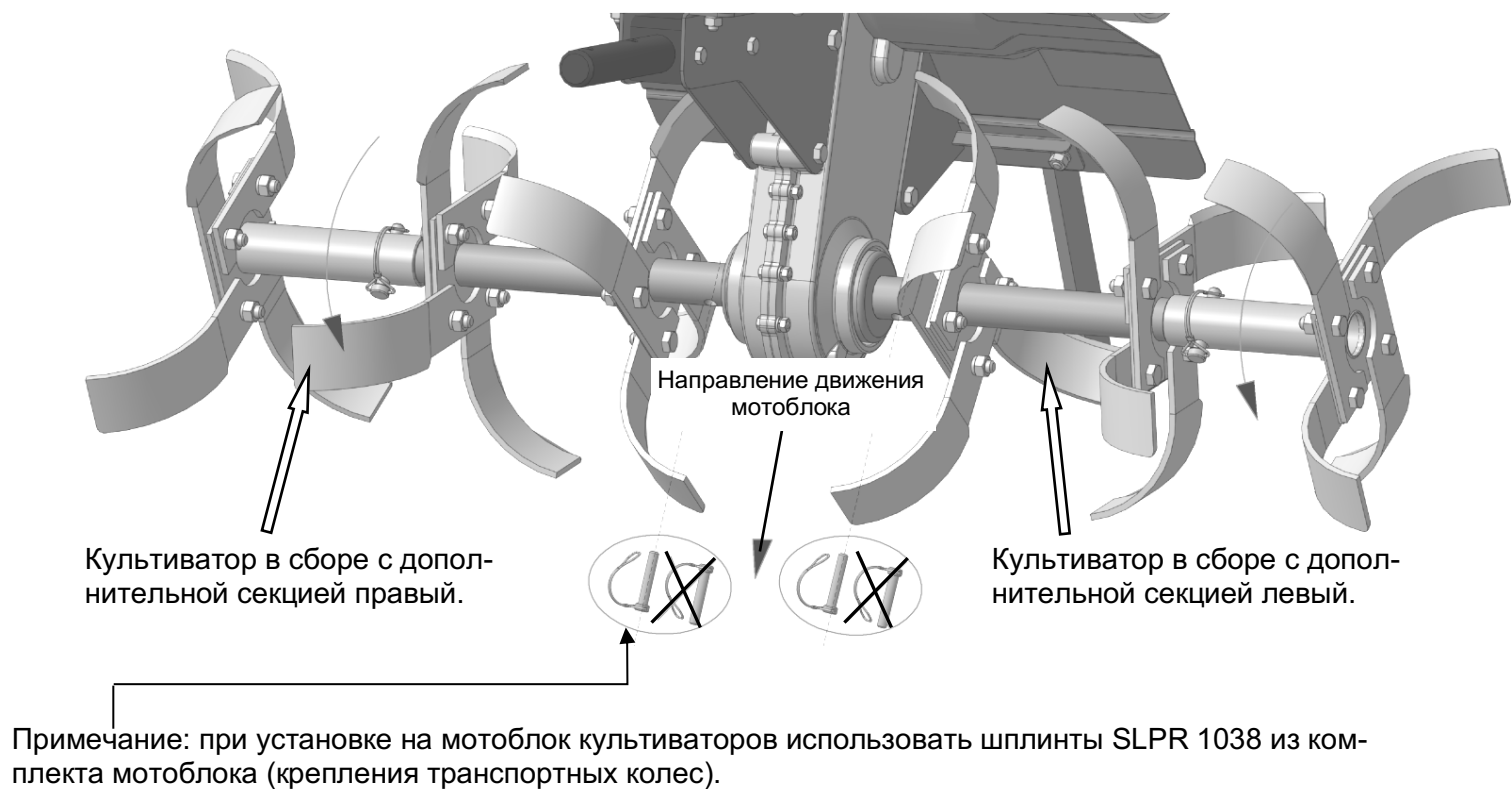
Рис.11. Схема сборки мотоблока с культиваторами - 6 секций. МКМ-3.
